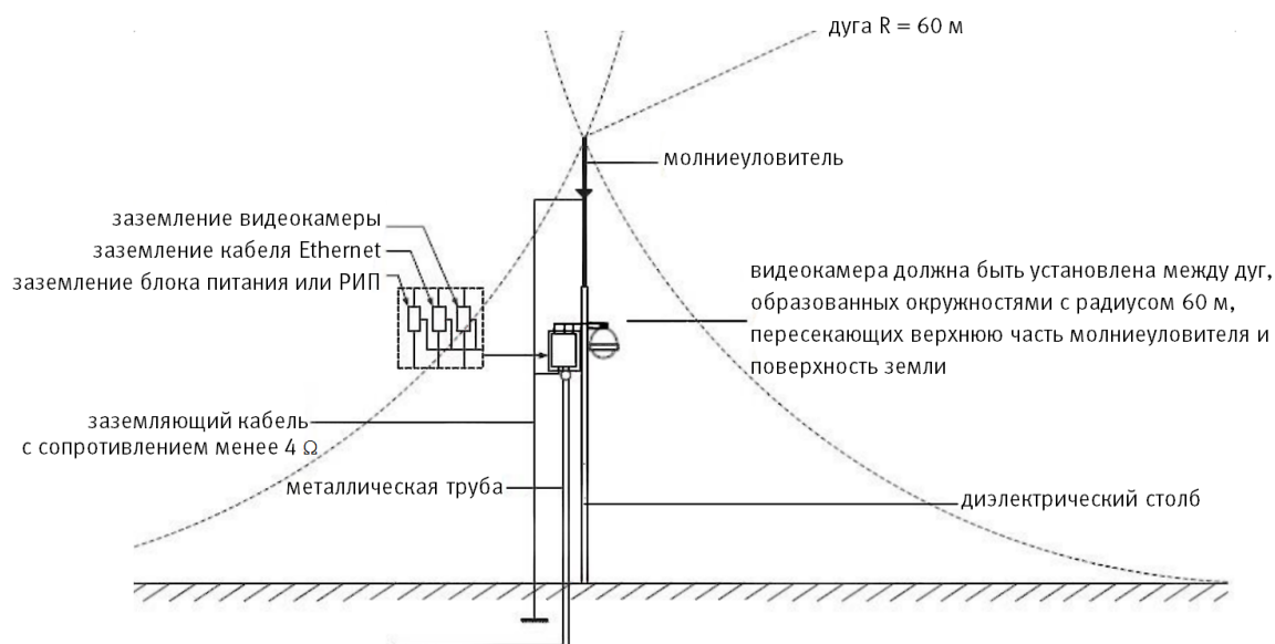
Рисунок 6.13 – Установка молниеотвода
