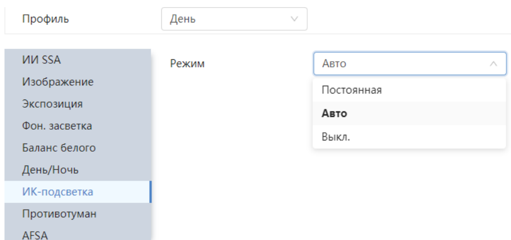
Рисунок 7.34 – Вкладка «Изображение: ИК-подсветка»
