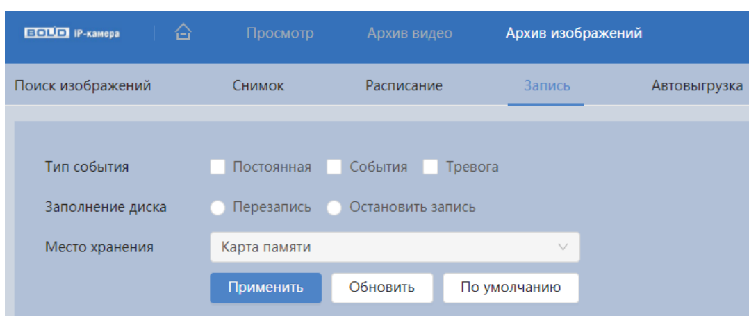
Рисунок 7.97 – Вкладка «Запись»
