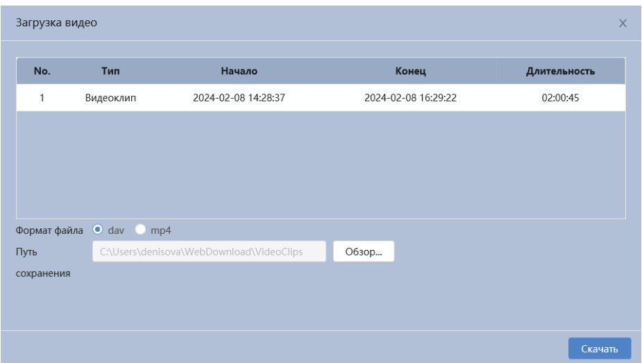
Рисунок 7.86 – Загрузка видео
