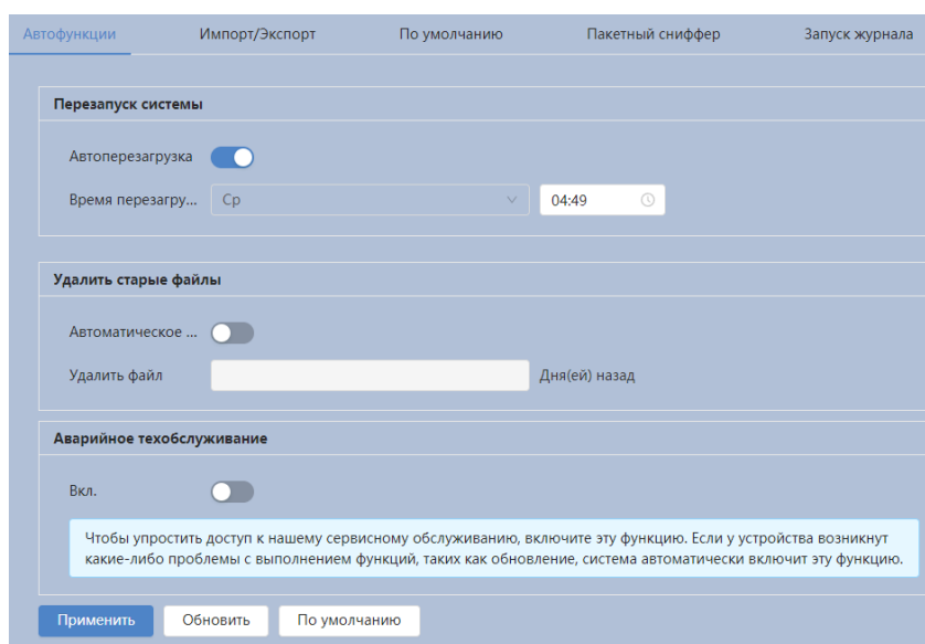
Рисунок 7.77 – Вкладка «Автофункции»
