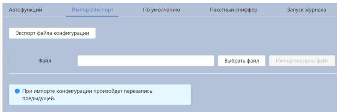
Рисунок 7.78 – Вкладка «Импорт/Экспорт»
