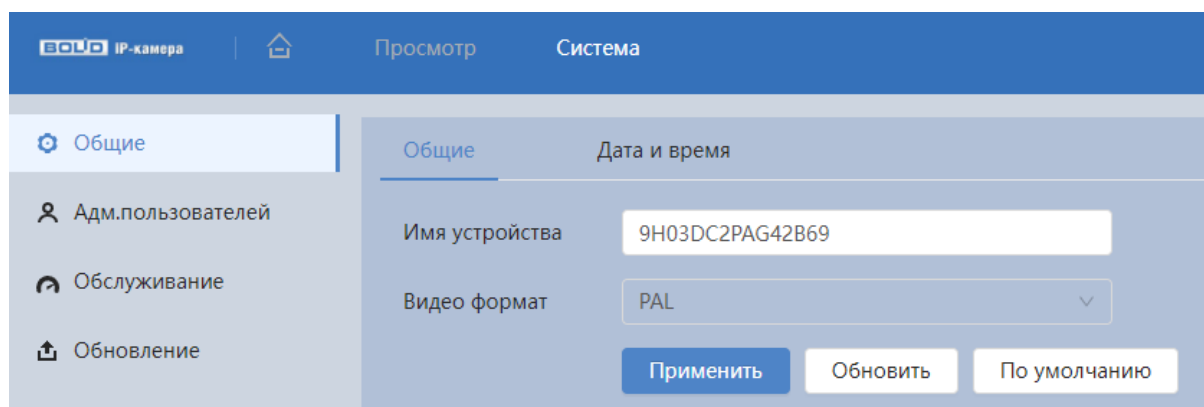
Рисунок 7.69 – Вкладка «Общие»
