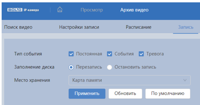
Рисунок 7.90 – Вкладка «Запись»
