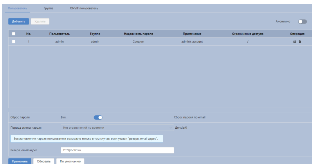
Рисунок 7.72 – Вкладка «Пользователь»
