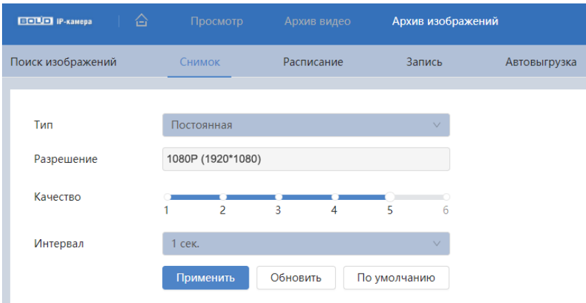
Рисунок 7.93 – Вкладка «Снимок»
