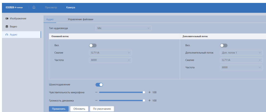
Рисунок 7.48 – Вкладка «Аудио»
