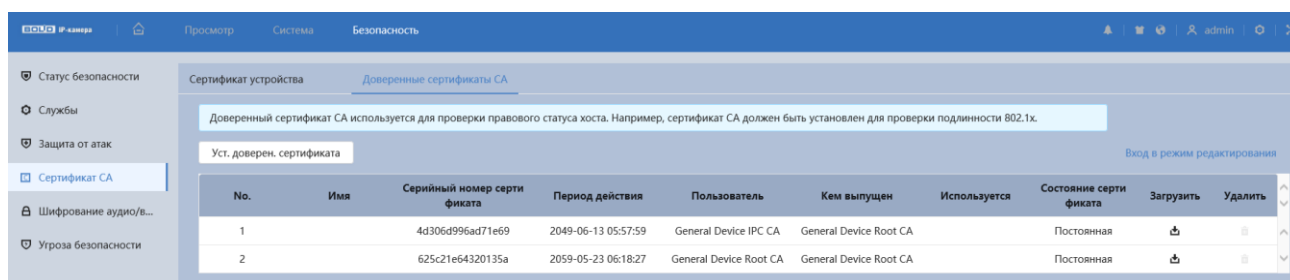
Рисунок 7.113 – Вкладка «Доверенные сертификаты CA»
