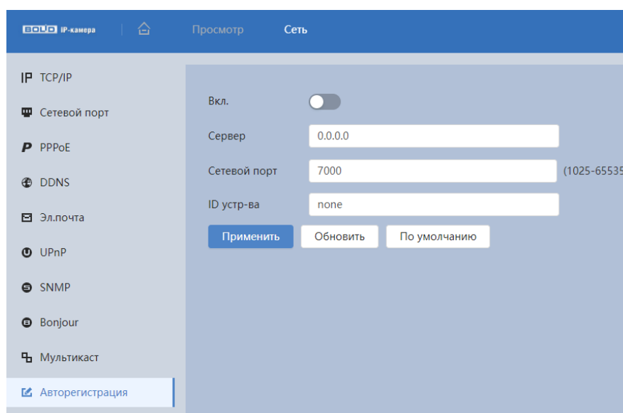
Рисунок 8.16 – Подпункт меню «Авторегистрация»
