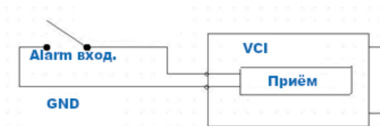
Рисунок 6.12 – Схема подключения тревожного входа
