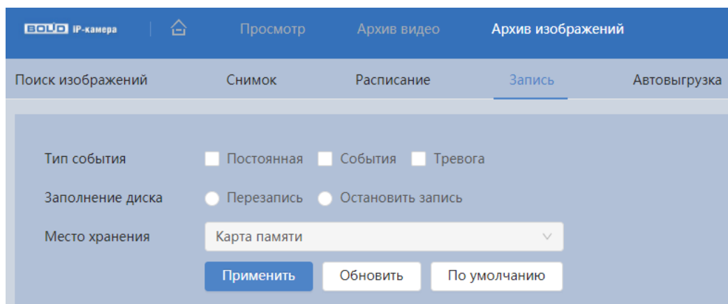
Рисунок 7.96 – Вкладка «Запись»
