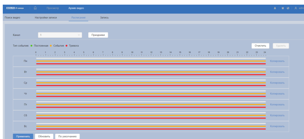
Рисунок 7.88 – Вкладка «Расписание»
