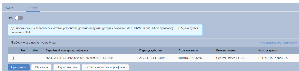
Рисунок 7.104 – Вкладка «HTTPS»
