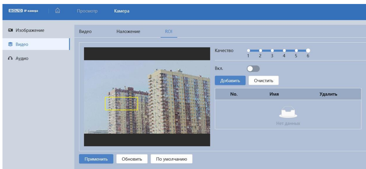
Рисунок 7.46 – Вкладка «ROI»
