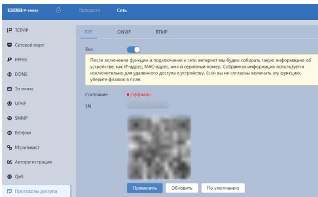
Рисунок 8.19 – Вкладка «P2P»
