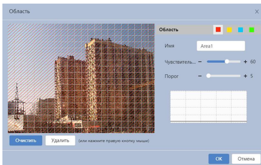
Рисунок 7.59 – Вкладка «Область»
