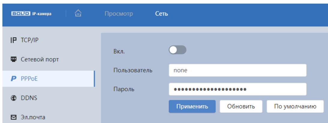
Рисунок 8.7 – Подпункт меню «PPPoE»
