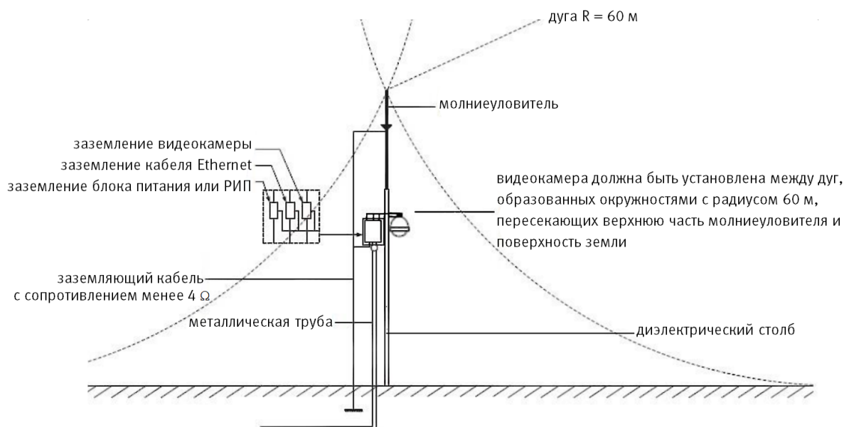
Рисунок 6.13 – Установка молниеотвода
