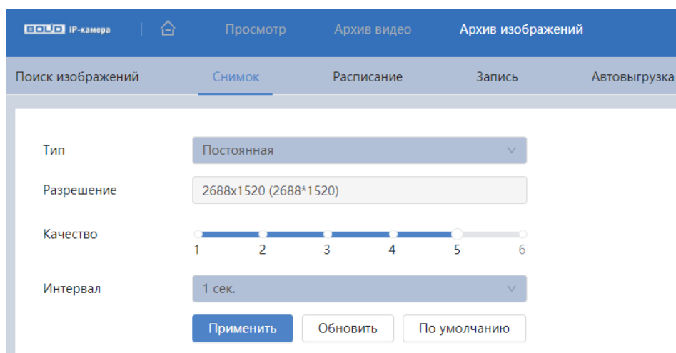
Рисунок 7.93 – Вкладка «Снимок»
