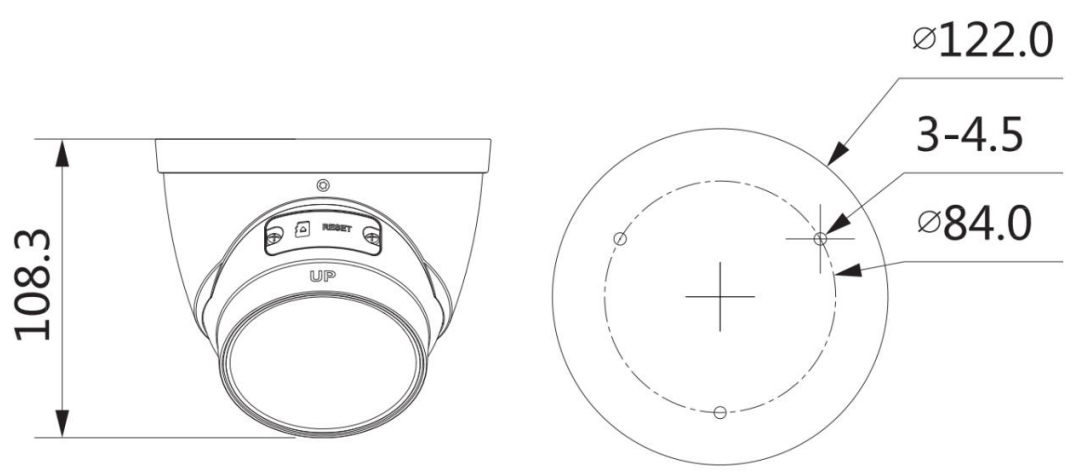
Рисунок 5.1 – Габаритные размеры видеокамеры
