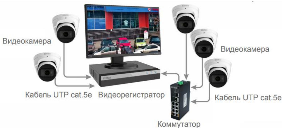
Рисунок 6.4 – Схема подключения видеокамеры к видеорегистратору
