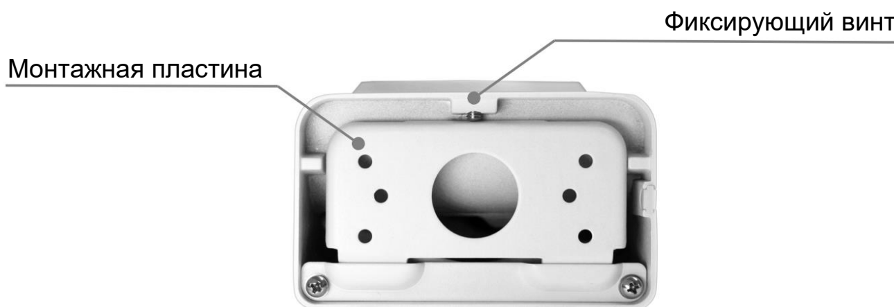
Рисунок 5.8 – Настенный кронштейн
