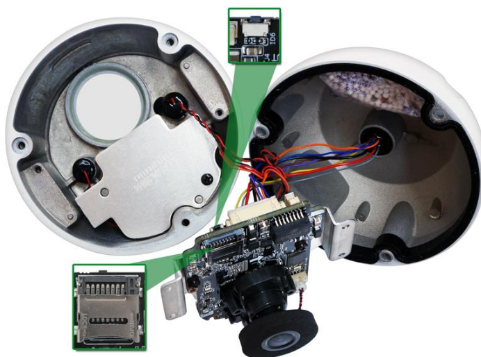
Рисунок 4.2 – Расположение кнопки аппаратного сброса и слота для карты памяти
