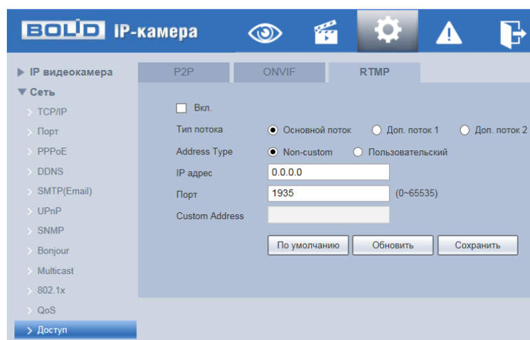
Рисунок 7.68 – Вкладка «RTMP»
