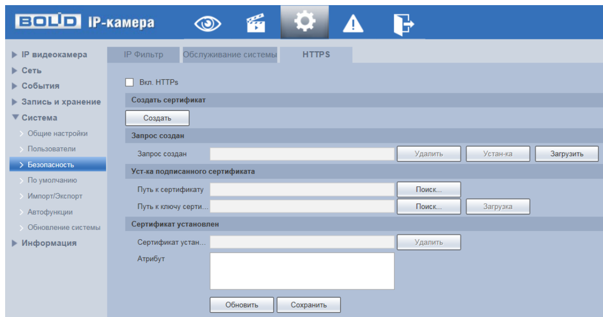
Рисунок 7.116 – Вкладка «HTTPS»
