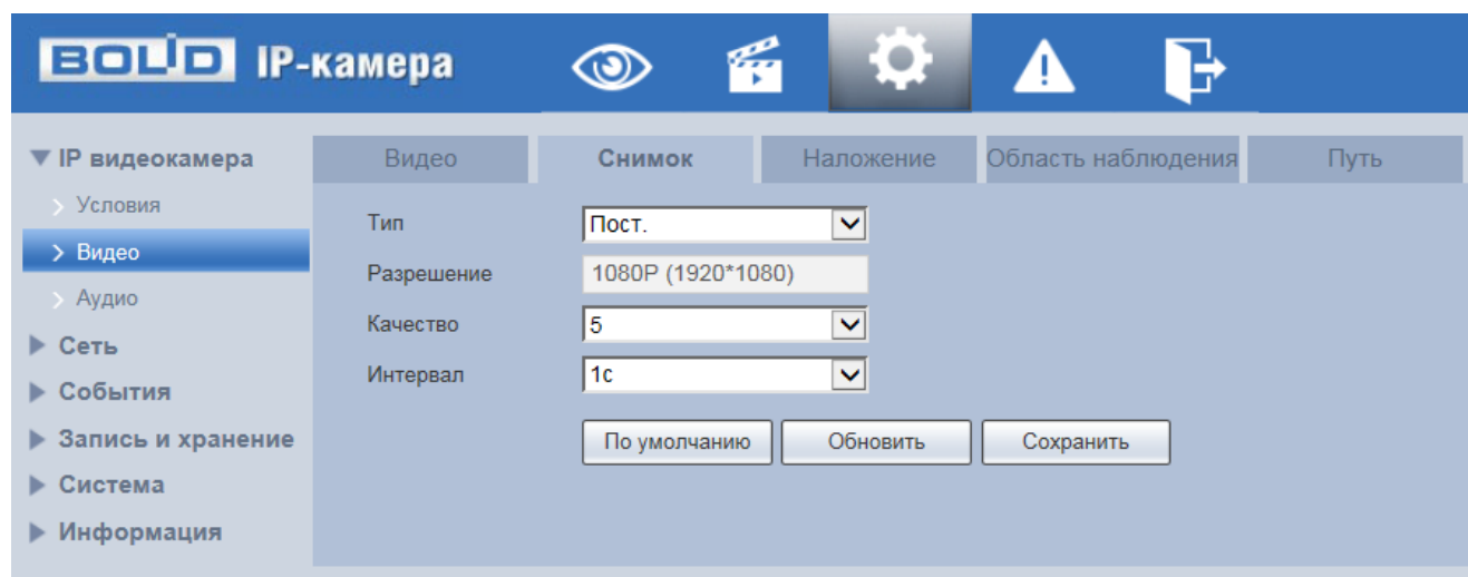
Рисунок 7.39 – Вкладка «Снимок»
