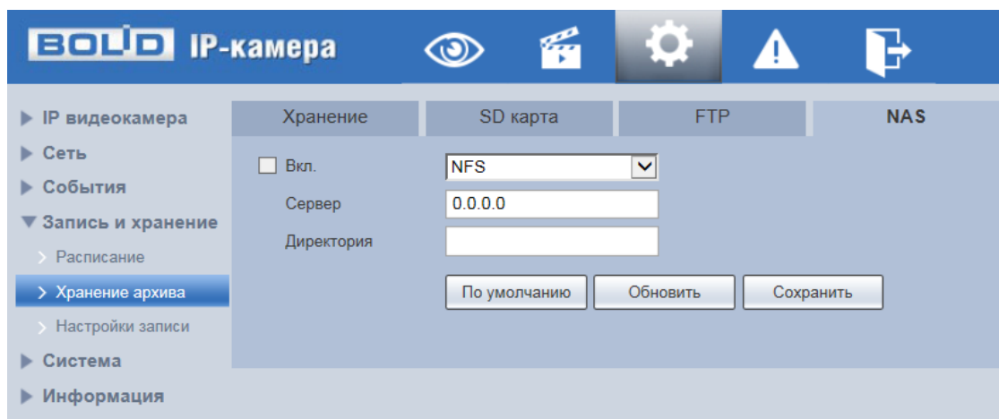
Рисунок 7.102 – Вкладка «NAS»
