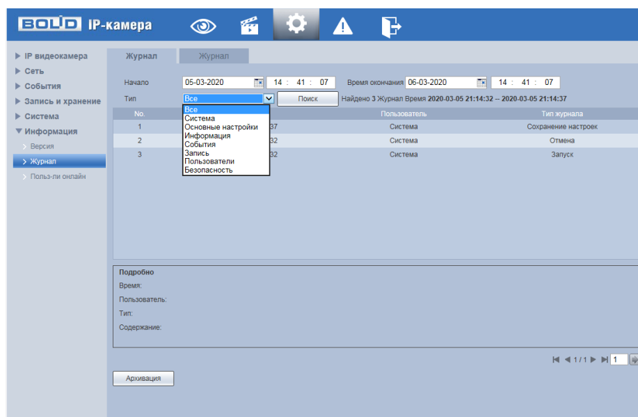
Рисунок 7.125 – Вкладка «Журнал»
