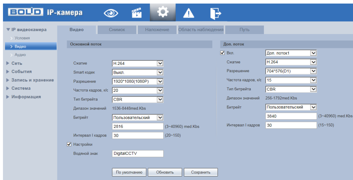
Рисунок 7.38 – Вкладка «Видео»
