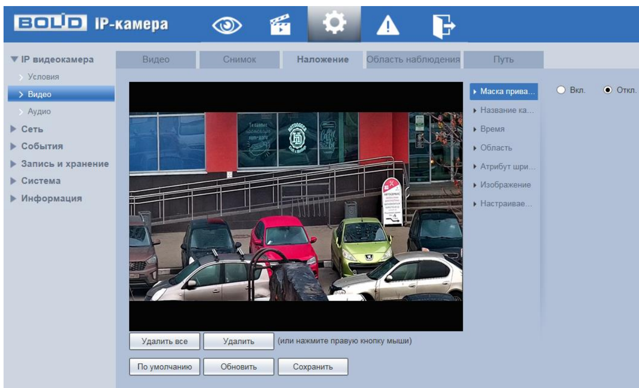
Рисунок 7.40 – Вкладка «Наложение»
