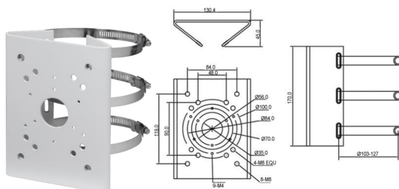
Рисунок 5.13 – Столбвой кронштейн BR-103
