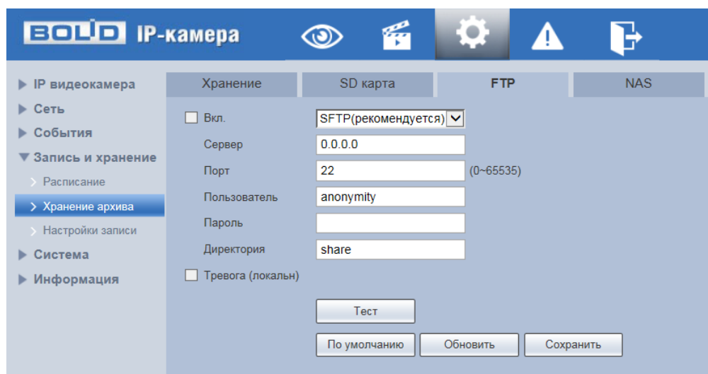
Рисунок 7.101 – Вкладка «FTP»
