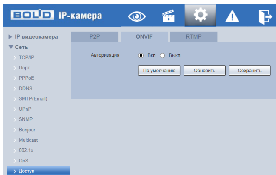
Рисунок 7.67 – Вкладка «ONVIF»
