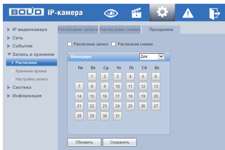
Рисунок 7.97 – Вкладка «Праздники»
