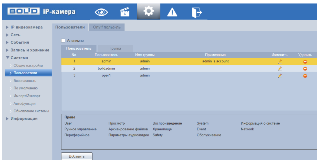
Рисунок 7.110 – Вкладка «Пользователи»
