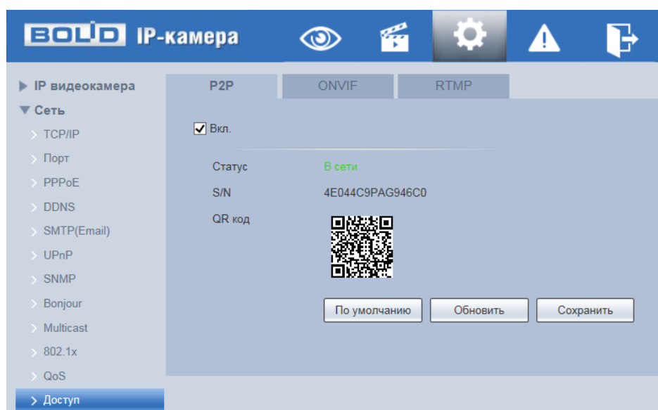
Рисунок 7.66 – Вкладка «P2P»
