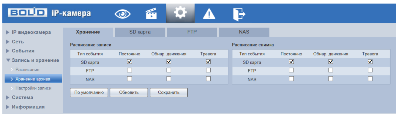
Рисунок 7.99 – Вкладка «Хранение»
