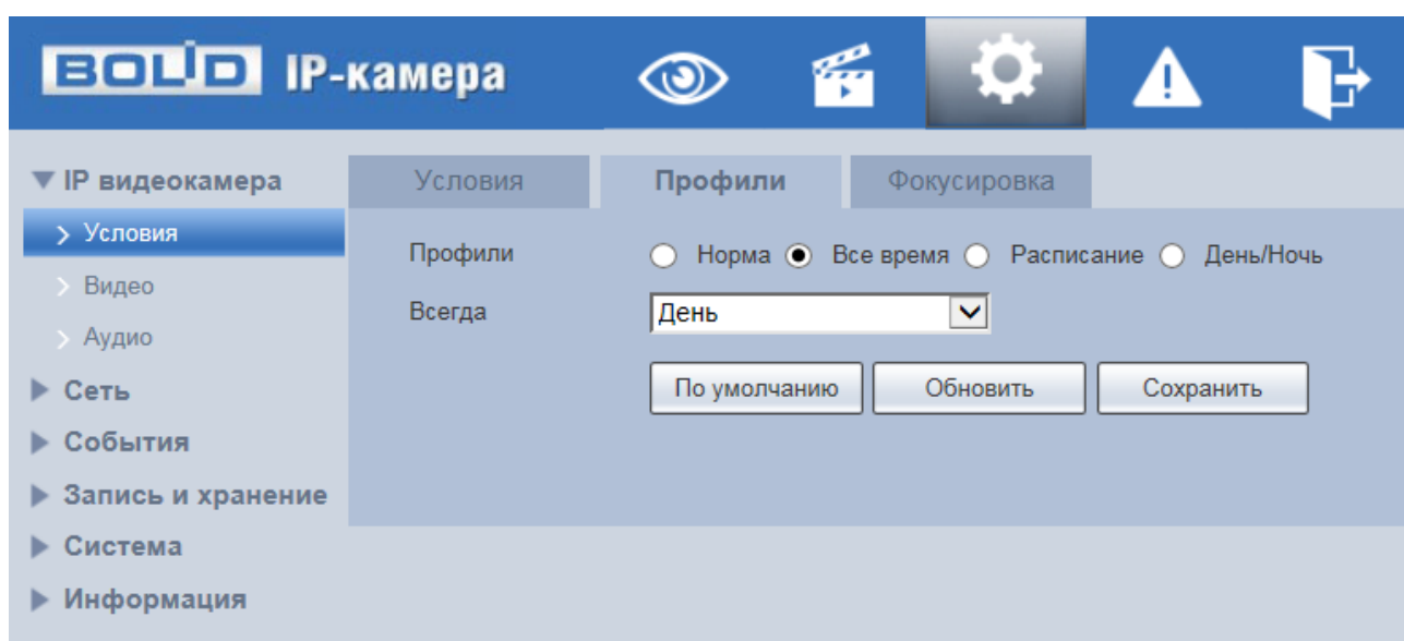
Рисунок 7.36 – Вкладка «Профили»
