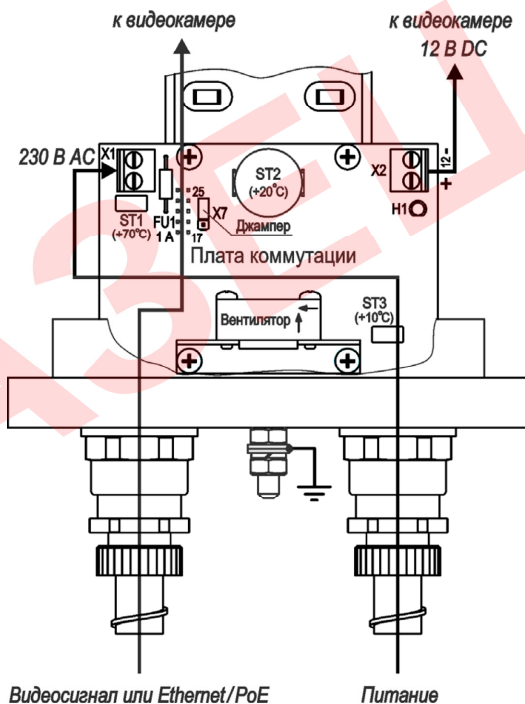
Рисунок 3 – Схема подключения IP-видеокмеры (220VAC)
