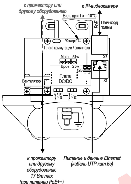
Рисунок 7 – Схема подключения ТВК-...-PoE++
