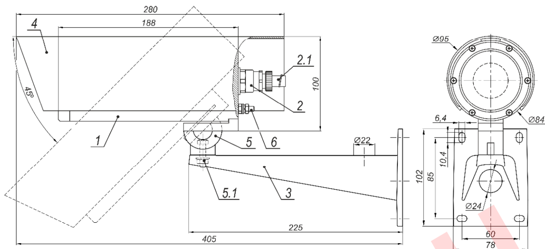
Рисунок 1 – Состав, габаритные и установочные размеры
