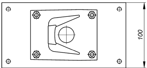
Крепление (вид спереди)
