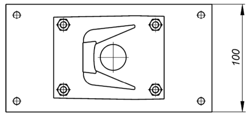
Крепление (вид спереди)
