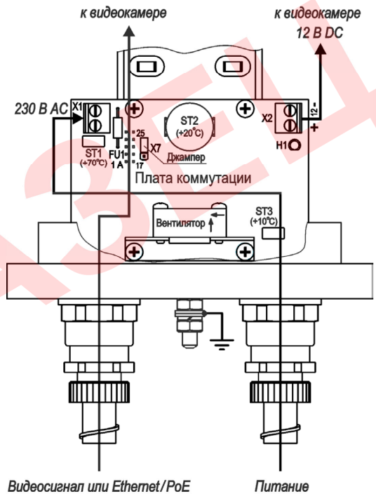
Рисунок 3 – Схема подключения IP-видеокамеры (220VAC)
