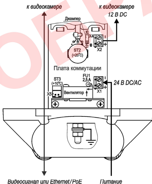
Рисунок 2 – Схема подключения IP-видеокамеры (24VDC/AC)
