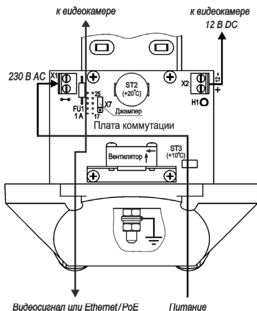
Рисунок 3 – Схема подключения IP-видеокамеры (220VAC)
