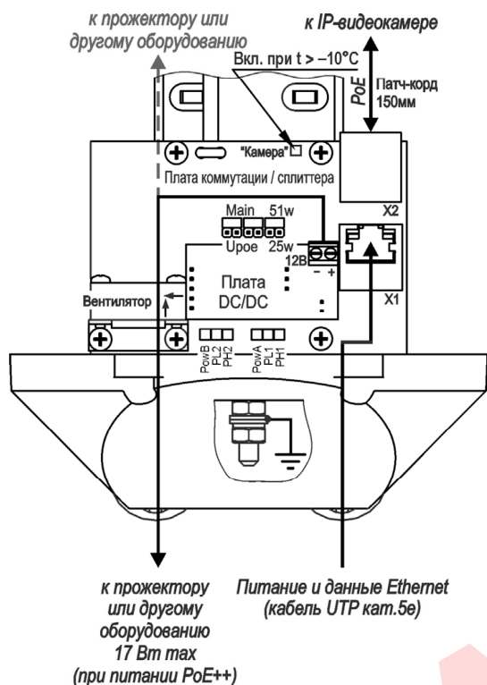
Рисунок 7 – Схема подключения ТВК-...-PoE++
