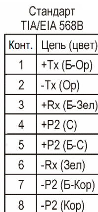
Рисунок 6 – Обжимка вилки RJ45 на кабель кат.5е
