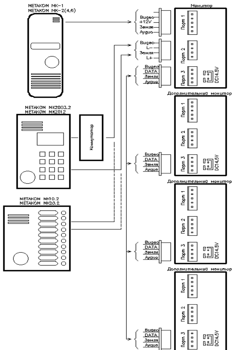
Рис. 3. Схема подключения видеомонитора МЕТАКОМ MKV-VM8 (вер. 2) в максимальной конфигурации.
