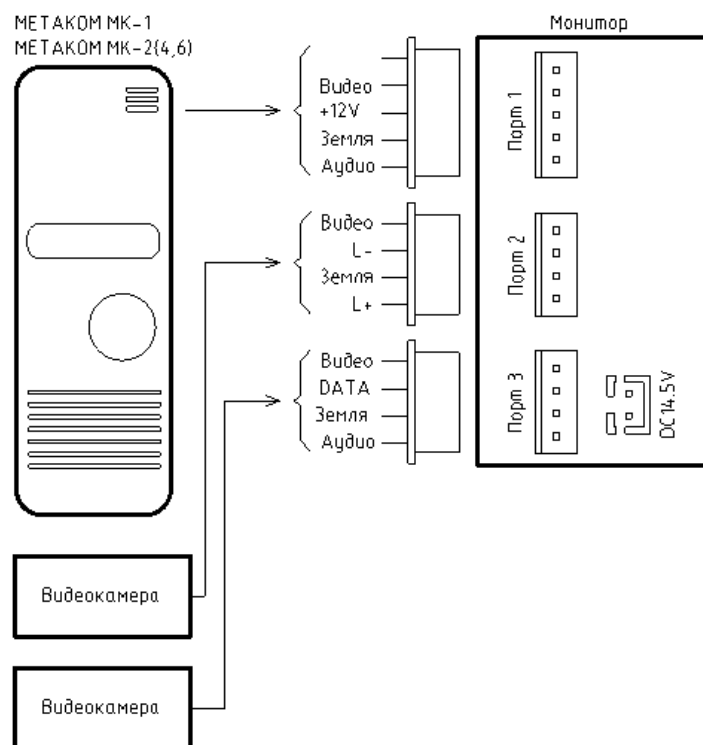
Рис. 4. Подключение дополнительных камер к видеомонитору МЕТАКОМ MKV-VM8 (вер. 2).
