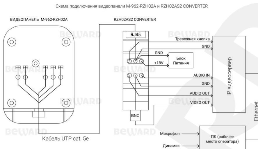
Рис. 3.4. Подключение конвертера к видеопанели
