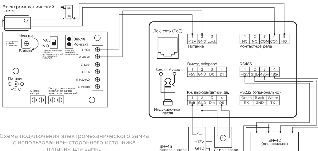
Схема подключения электрохимического замка с использованием блока бесперебойного питания UPS-DP/F
