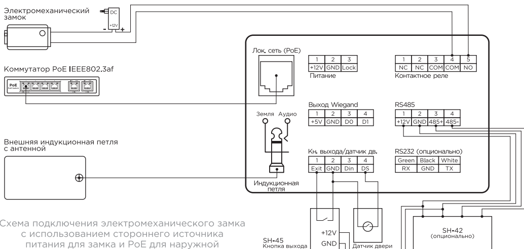
Схема подключения электрохимического замка с использованием стороннего источника питания для замка
