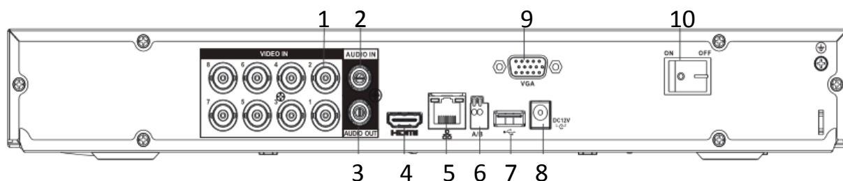
Рисунок 2 Задняя панель.
