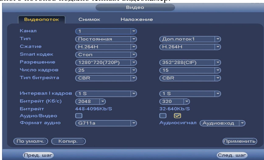
Рисунок 7 Интерфейс настройки видеопотоков
