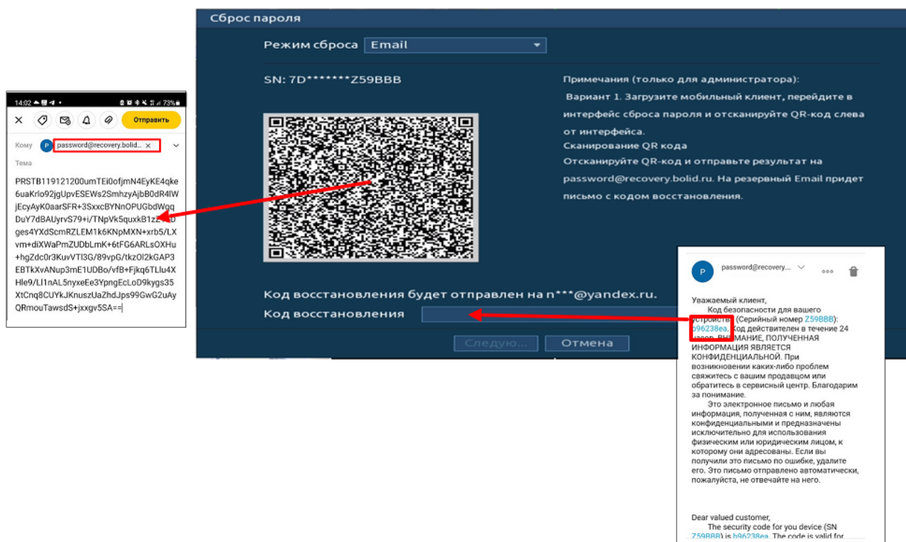
Рисунок 7.2 – Шаг 2. Восстановление пароля при помощи почты
