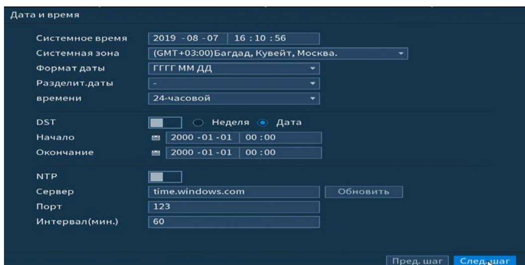
Рисунок 4.7 – Интерфейс настройки даты и времени Функции и диапазоны значений параметров даны в таблице ниже (Таблица 4.2).
