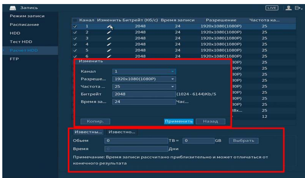
Рисунок 6.91 – Расчет времени
