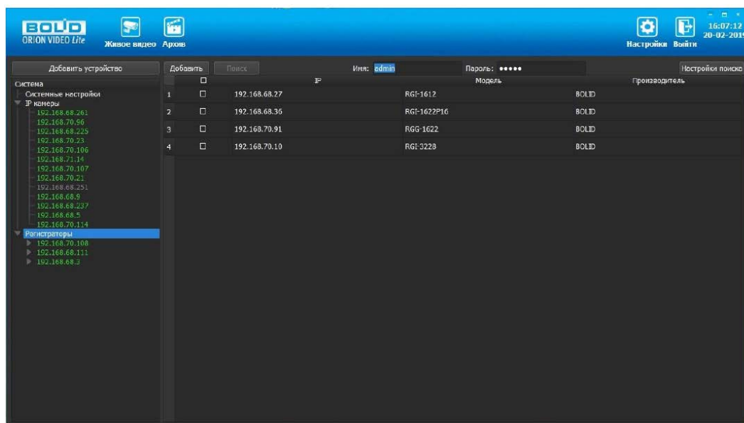
Рисунок 11.4 – Таблица результатов
