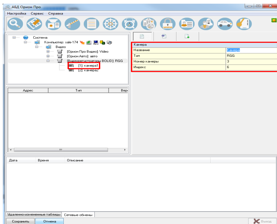
Рисунок 12.3 – Добавление камер
