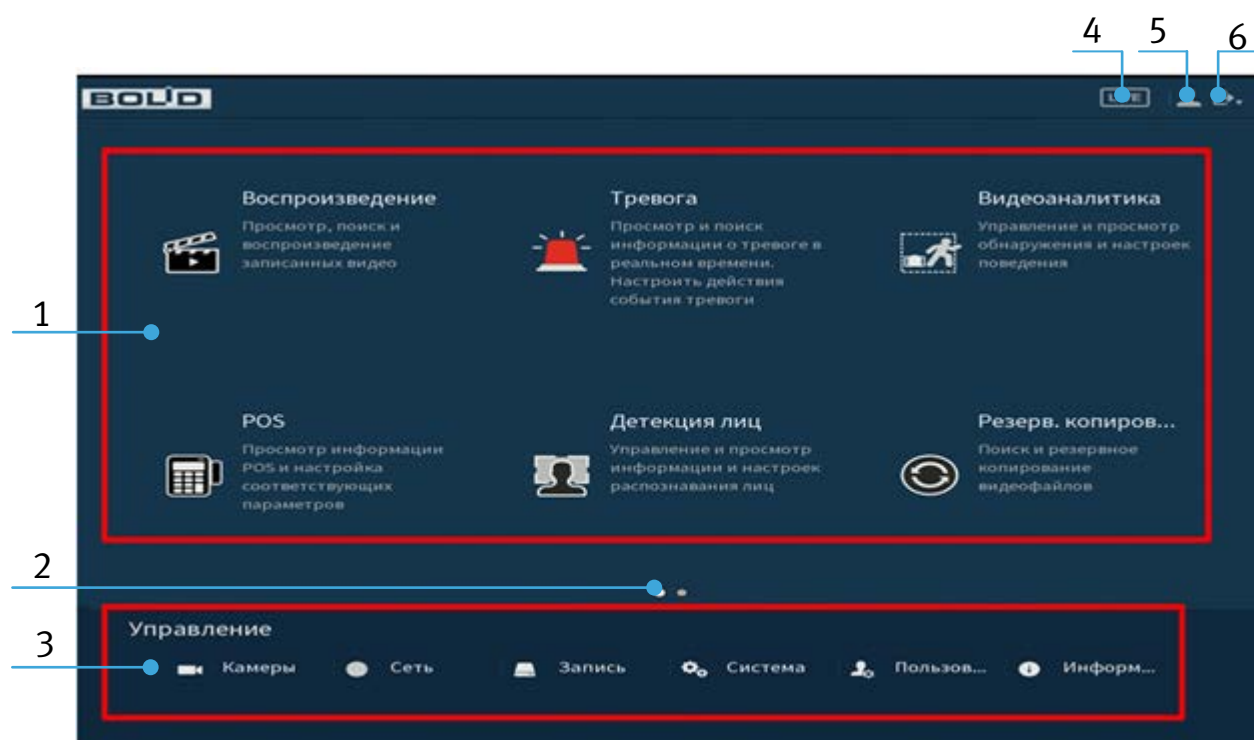
Рисунок 6.1 – Главное меню
