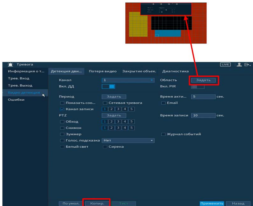
Рисунок 6.18 – Настройка области
