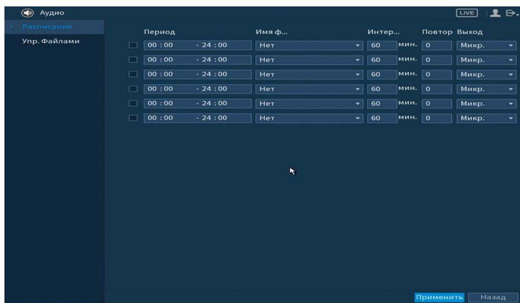
Рисунок 6.52 – Установка расписания
