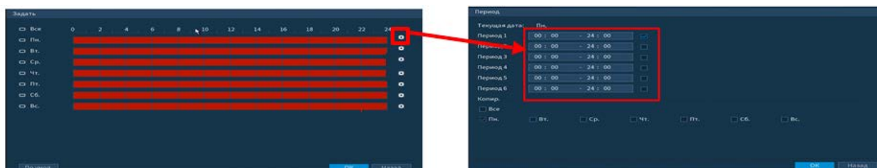
Рисунок 6.29 – Настройка расписания
