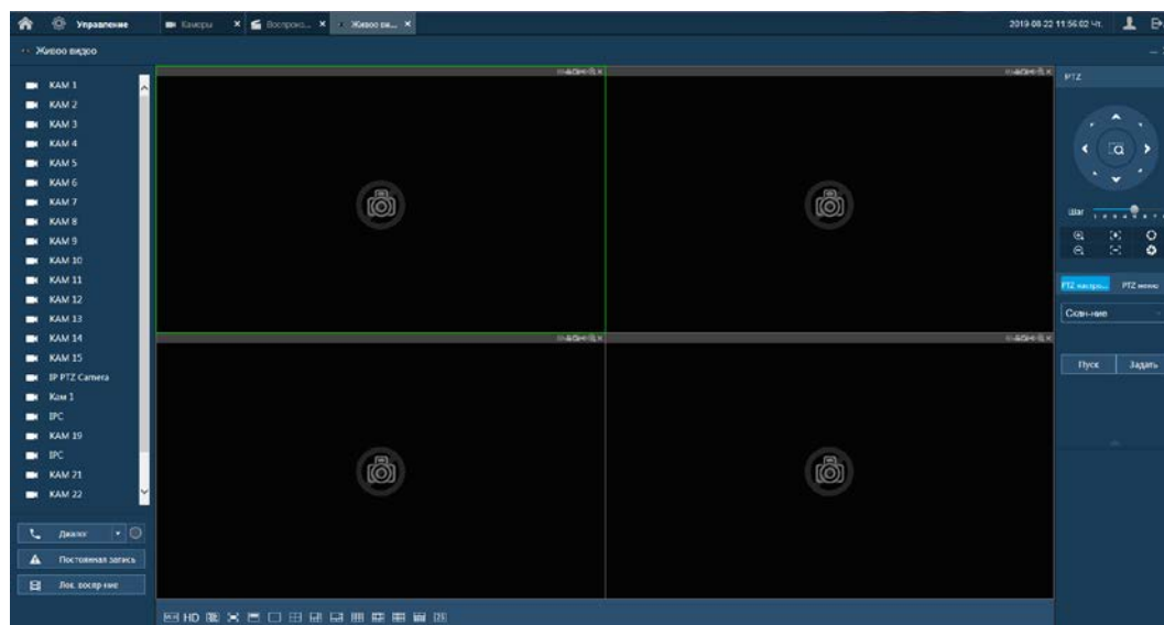
Рисунок 10.2 – Режим просмотра
