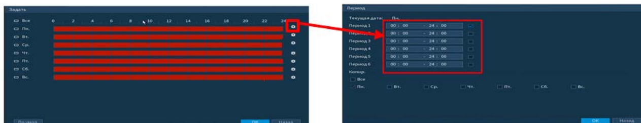
Рисунок 6.32 – Настройка расписания
