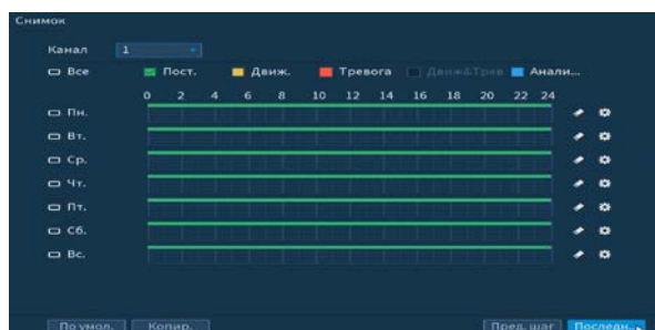
Рисунок 4.18 – Настройка расписания
