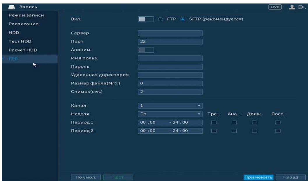
Рисунок 6.93 – Настройка FTP
