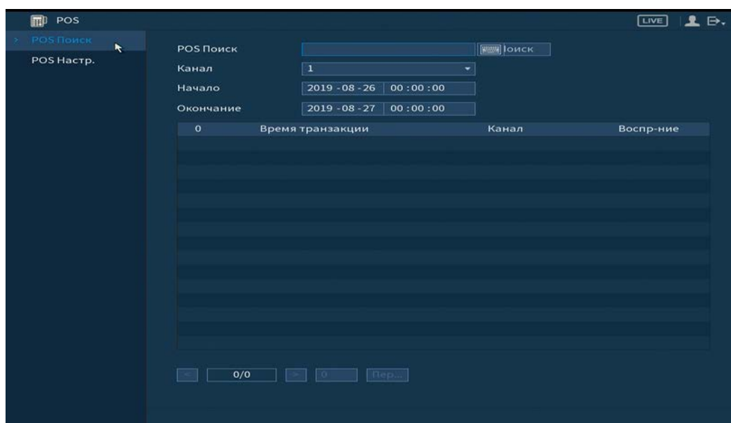
Рисунок 6.40 – Интерфейс поиска
