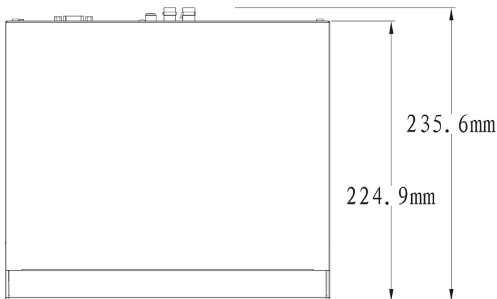
Рисунок 3.9 – Габаритные размеры видеорегистратора
