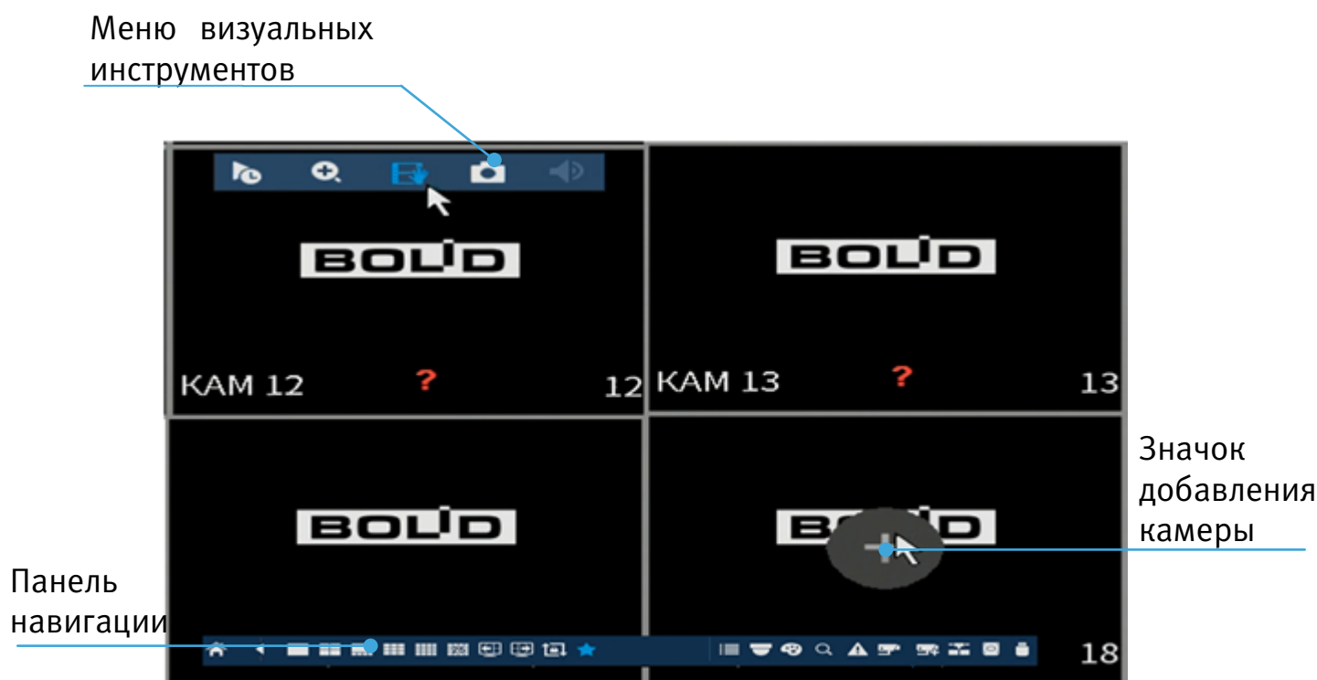
Рисунок 5.10 – Добавление IP-камер
