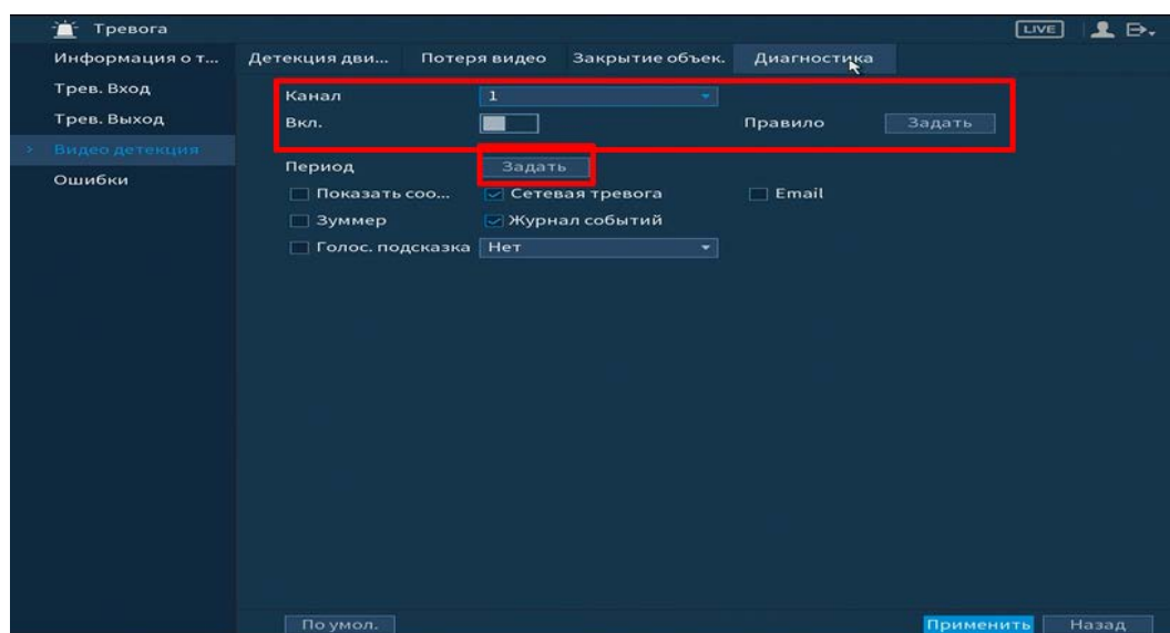
Рисунок 6.21 – Диагностика
