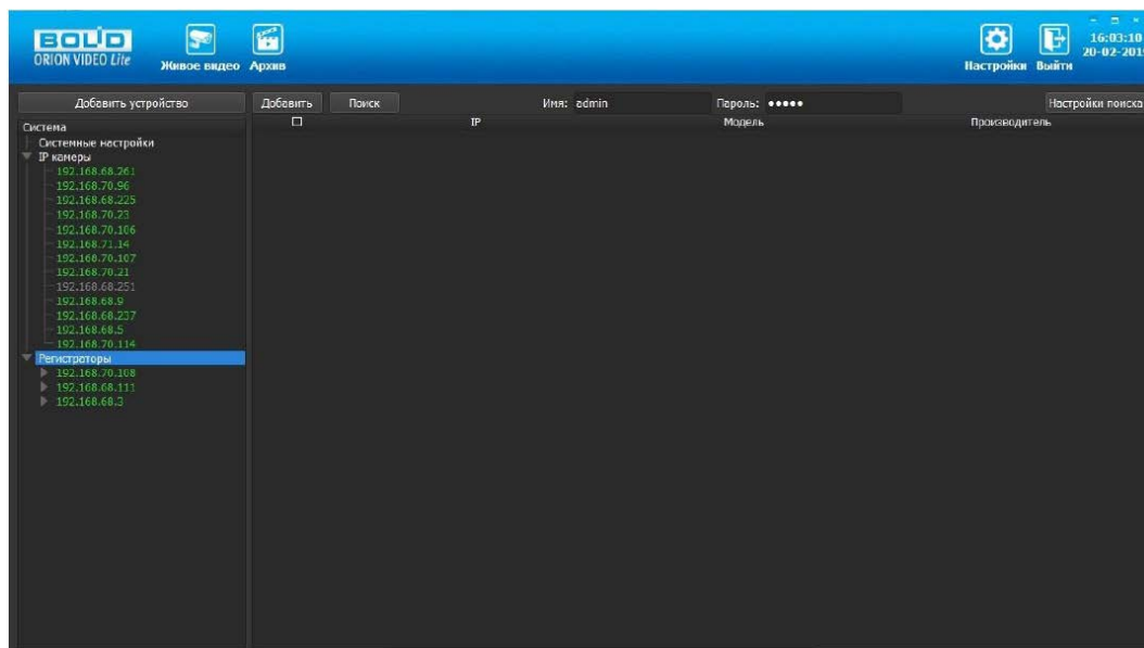
Рисунок 11.2 – Поиск устройства
