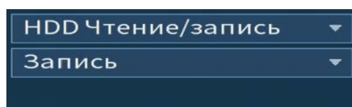
Рисунок 6.7 – Тип поиска
