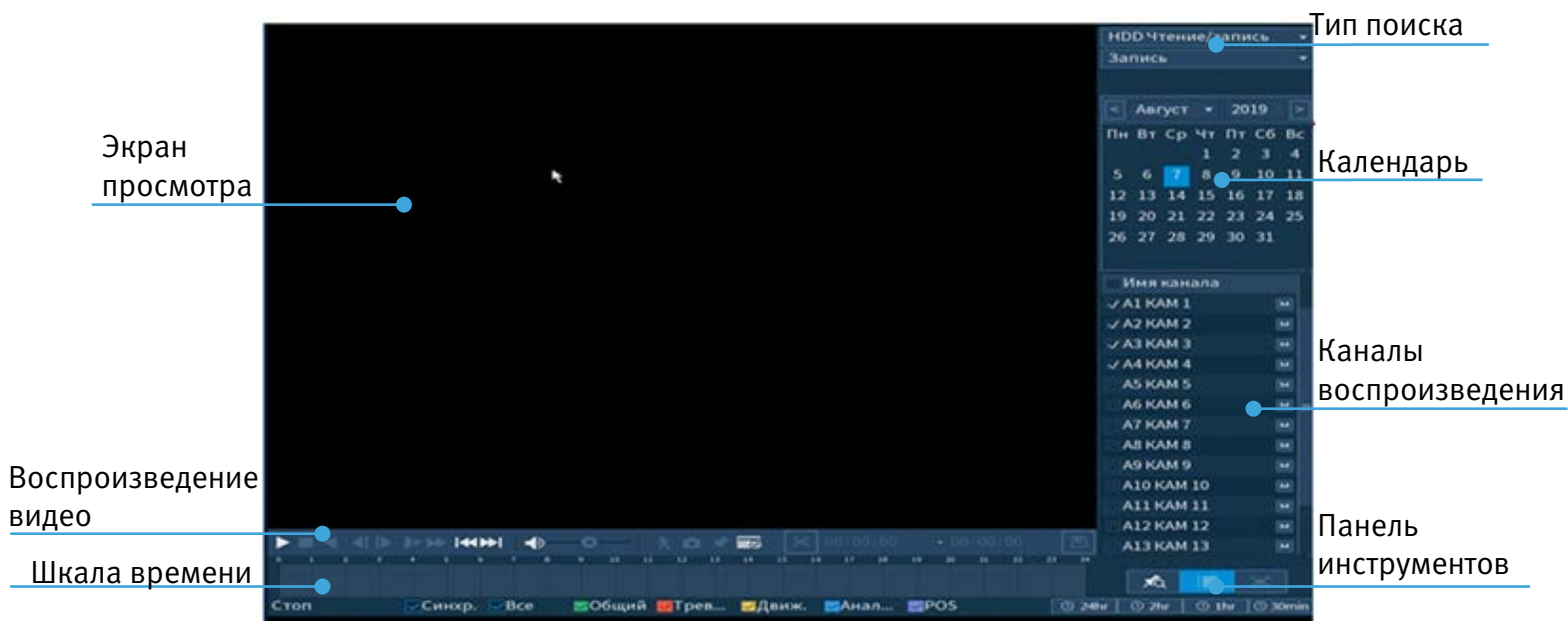
Рисунок 6.2 – Просмотр архива
