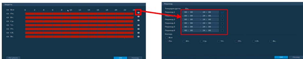
Рисунок 6.35 – Настройка расписания
