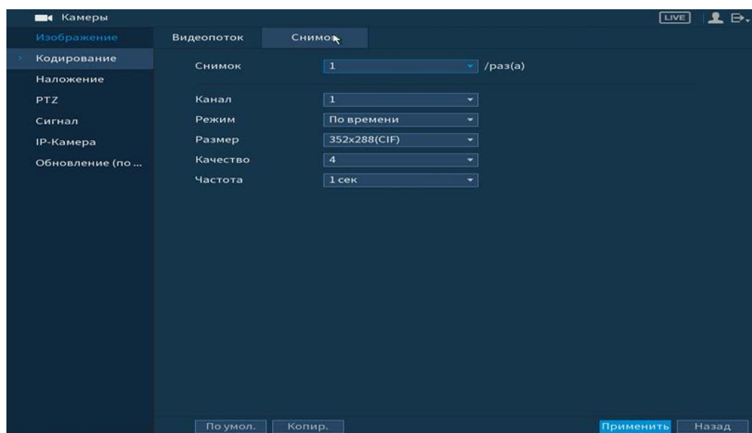
Рисунок 6.57 – Настройка снимка
