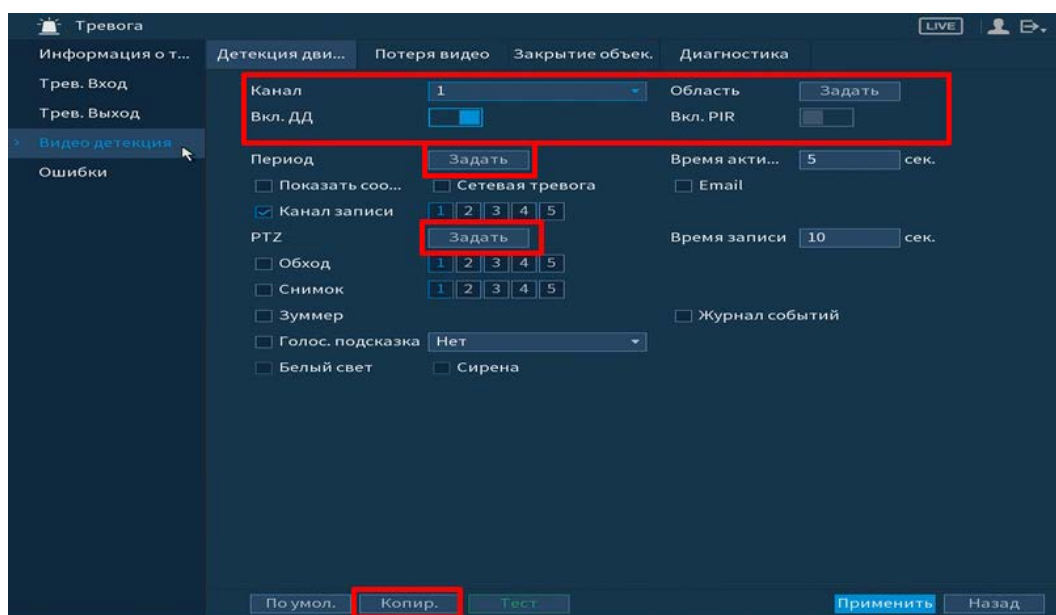
Рисунок 6.17 – Настройка события
