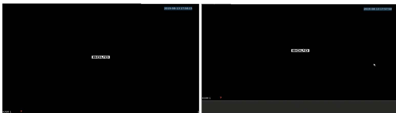
Рисунок 5.14 – Варианты просмотра
