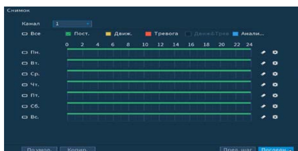
Рисунок 4.15 – Настройка расписания
