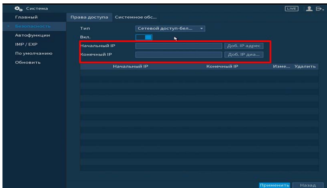
Рисунок 6.97 – Права доступа
