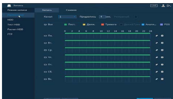
Рисунок 6.83 – Настройка расписания
