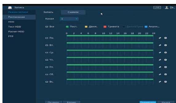
Рисунок 6.86 – Настройка расписания
