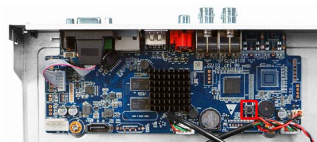
Рисунок 7.10 – Кнопка сброса
