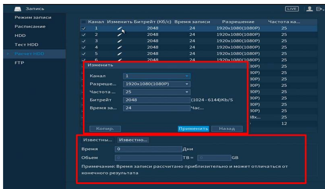
Рисунок 6.92 – Расчет объема
