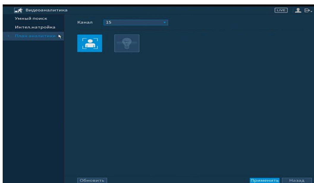
Рисунок 6.39 – Выбор функции
