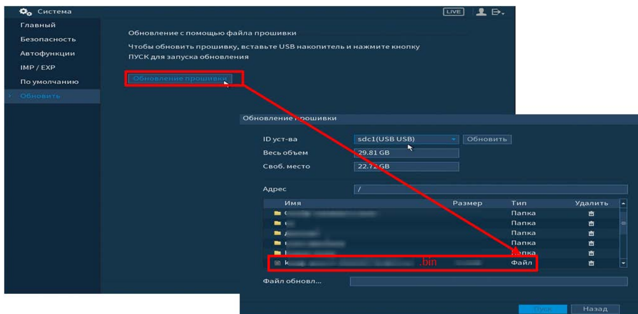
Рисунок 6.107 – Выбор файла для обновления
