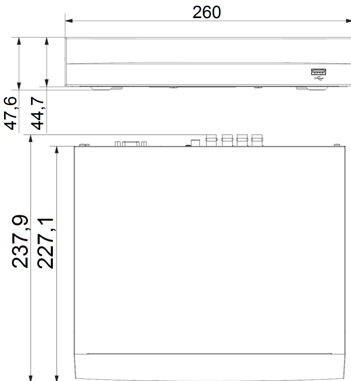
Рисунок 4.2 – Габаритные размеры
