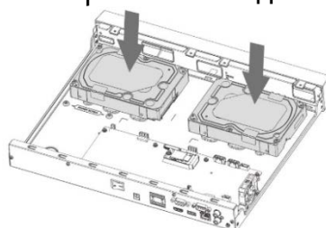
Рисунок 3.5 – Установка жесткого диска
