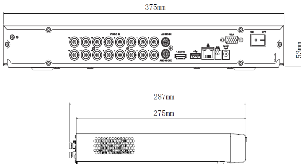
Рисунок 3.9 – Габаритные размеры видеорегистратора
