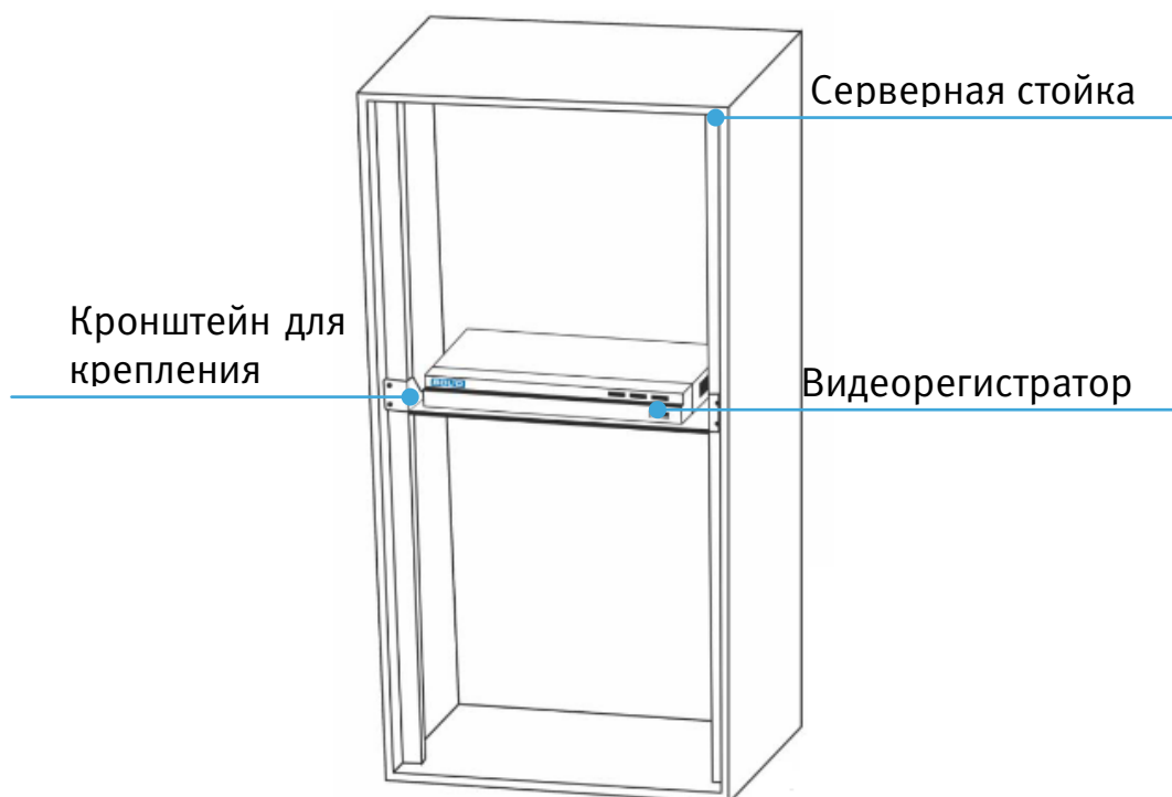
Рисунок 3.12 – Монтаж видеорегистратора в 19"- стойку с помощью кронштейна
