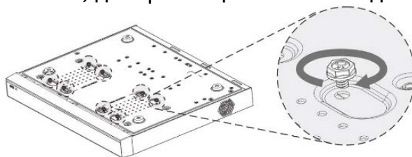
Рисунок 3.6 – Установка жесткого диска
