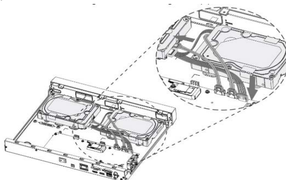
Рисунок 3.7 – Установка жесткого диска
