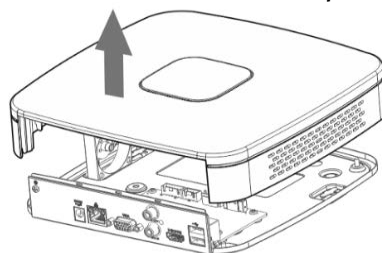
Рисунок 3.4 – Установка жесткого диска
