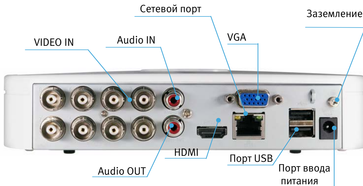
Рисунок 3.2 – Внешний вид задней панели
