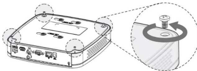
Рисунок 3.3 – Установка жесткого диска
