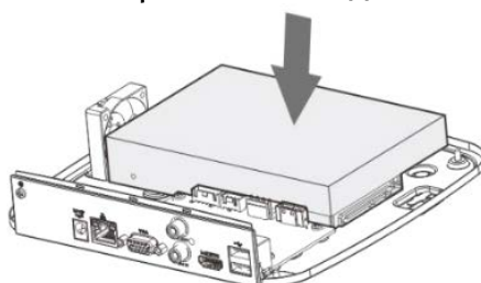
Рисунок 3.5 – Установка жесткого диска
