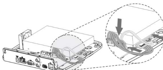
Рисунок 3.7 – Установка жесткого диска
