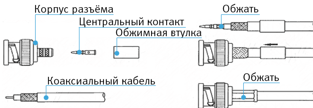
Рисунок 3.10 – Схема обжима BNC
