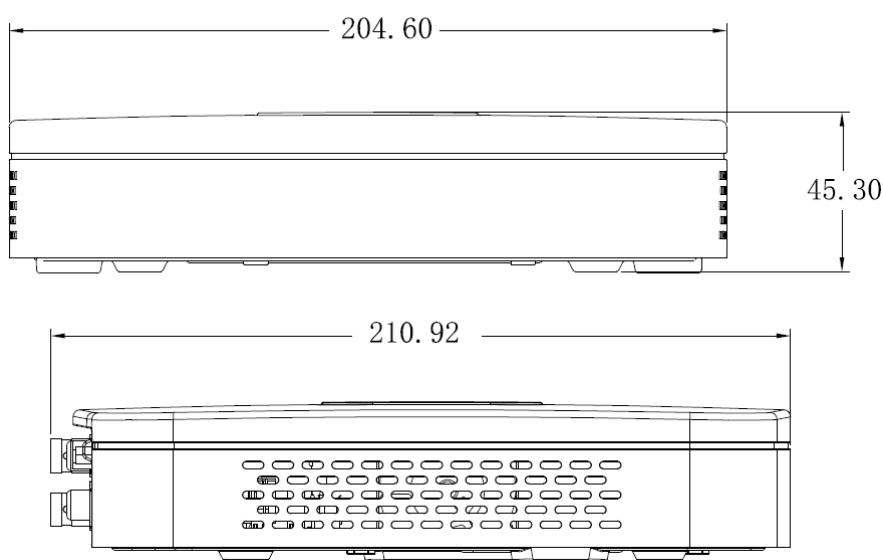
Рисунок 3.9 – Габаритные размеры видеорегистратора
