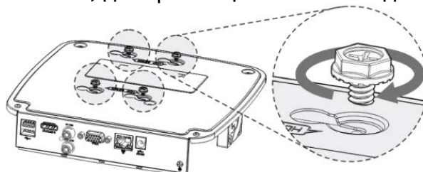
Рисунок 3.6 – Установка жесткого диска
