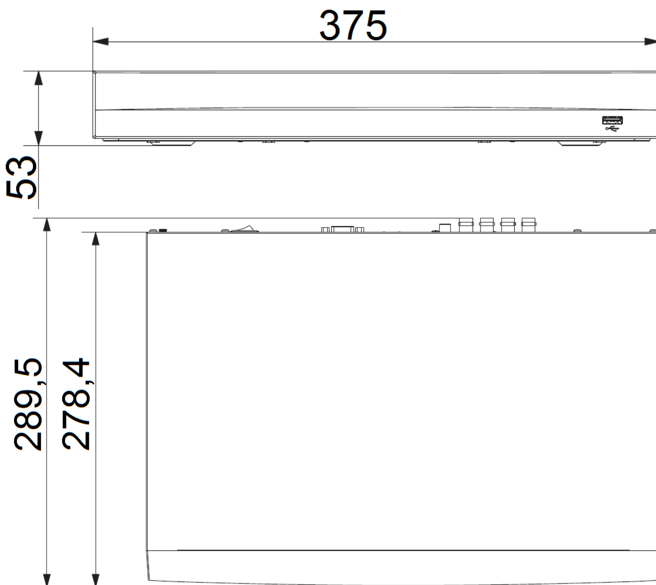
Рисунок 4.2 – Габаритные размеры
