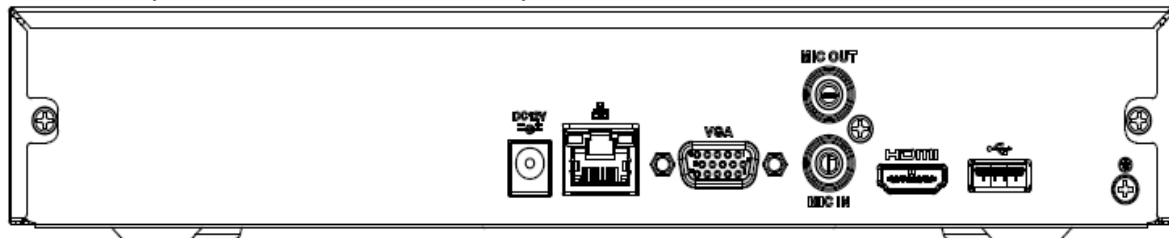
Рисунок 1.7 – Внешний вид задней панели корпуса
