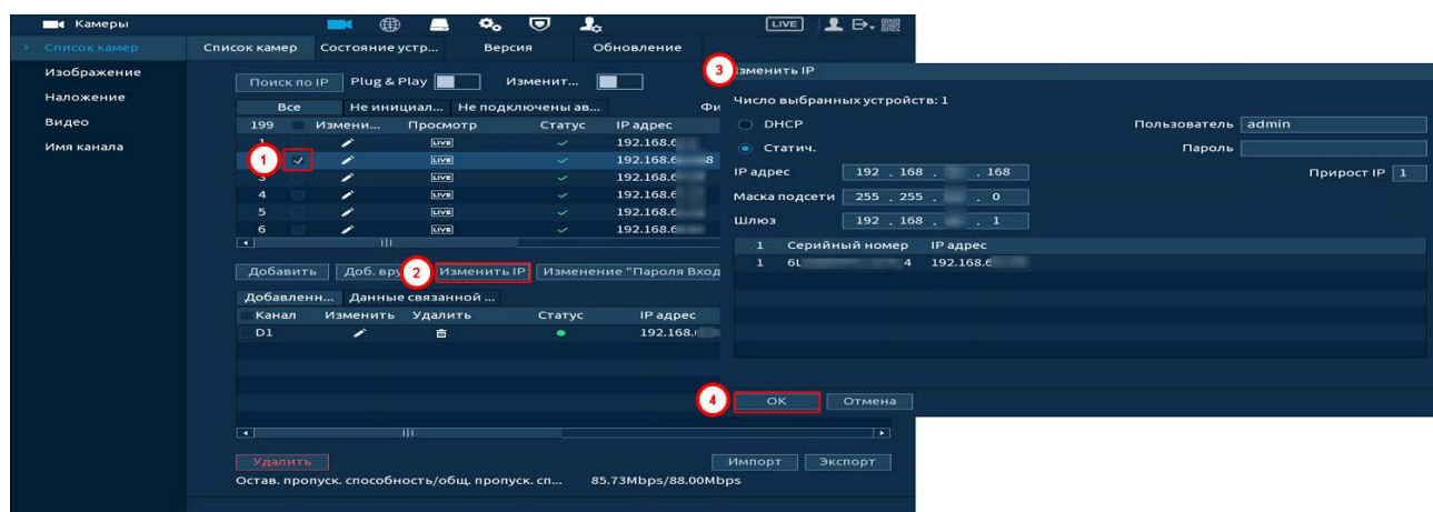
Рисунок 11.20 – Изменения сетевых настроек IP-камер через регистратор
