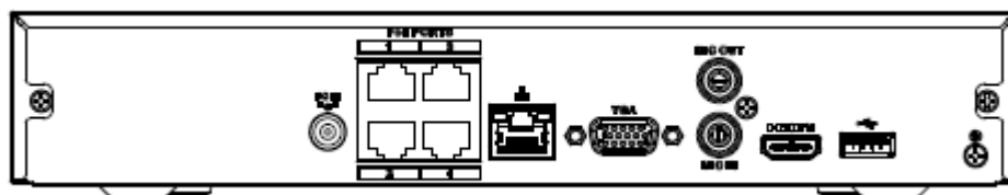
Рисунок 1.7 – Внешний вид задней панели корпуса
