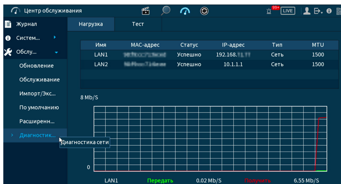
Рисунок 18.21 – Интерфейс просмотра нагрузки
