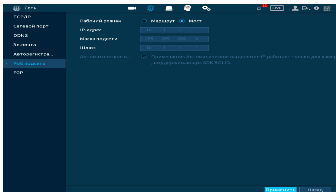
Рисунок 12.8 – Интерфейс настройки «РоЕ подсеть»
