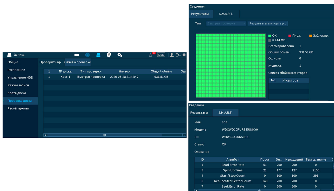
Рисунок 13.19 – Просмотр информации о HDD
