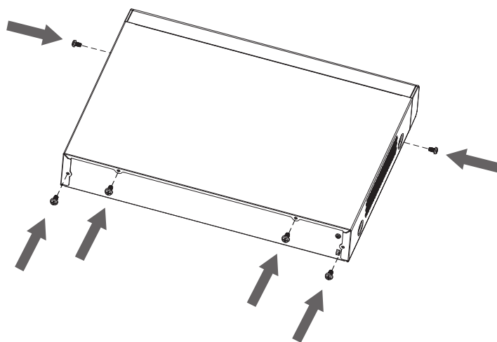
Рисунок 4.6 – Установка жёсткого диска
