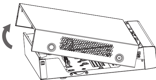
Рисунок 4.3 – Установка жёсткого диска
