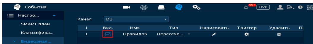
Рисунок 14.39 – Настройка
