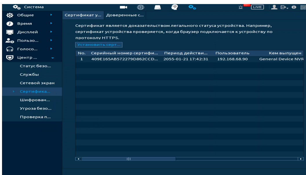
Рисунок 17.50 – Сертификат устройства
