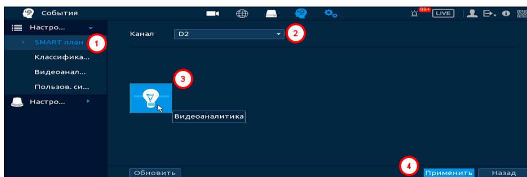
Рисунок 14.47 – Настройка
