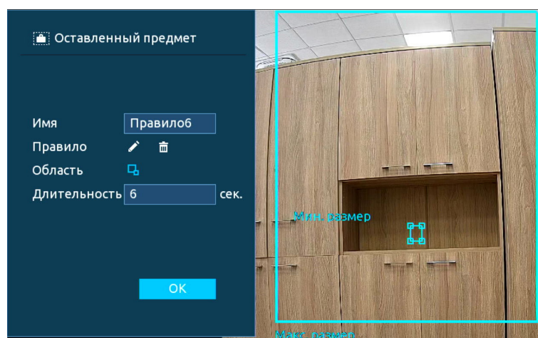
Рисунок 14.62 – Настройка функции
