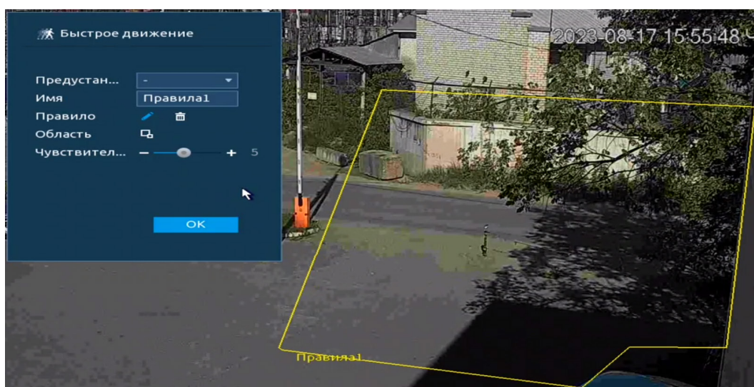
Рисунок 14.80 – Настройка правила
