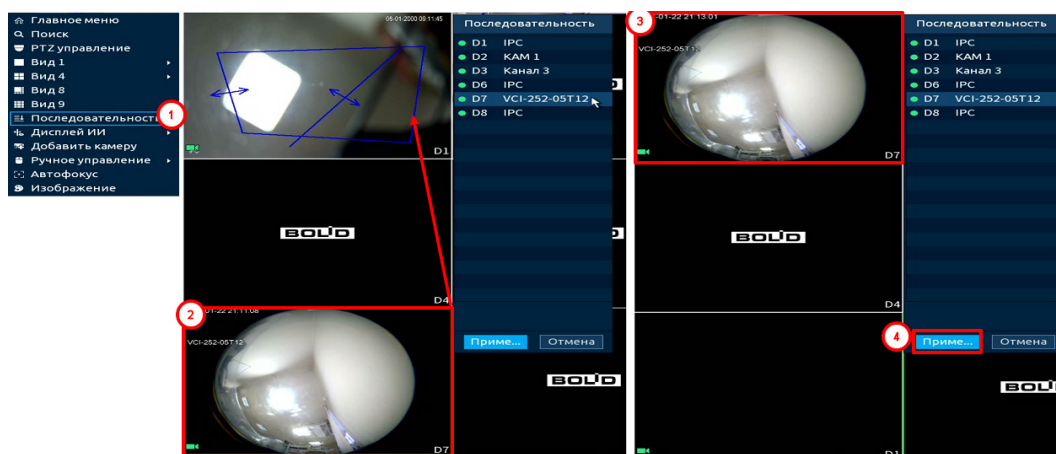
Рисунок 8.7 – Изменение раскладки
