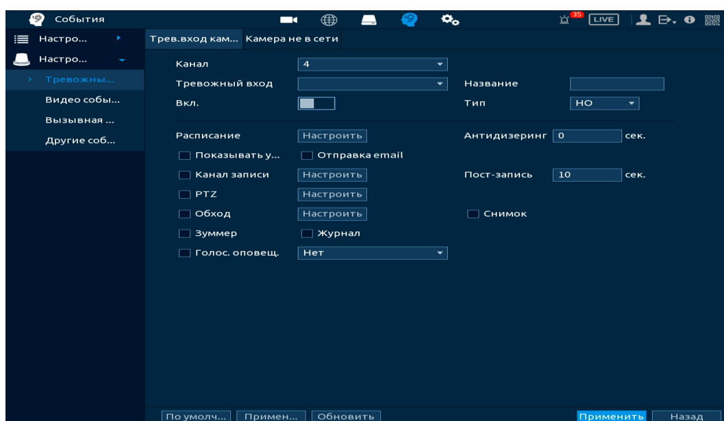
Рисунок 14.1 – Интерфейс настройки
