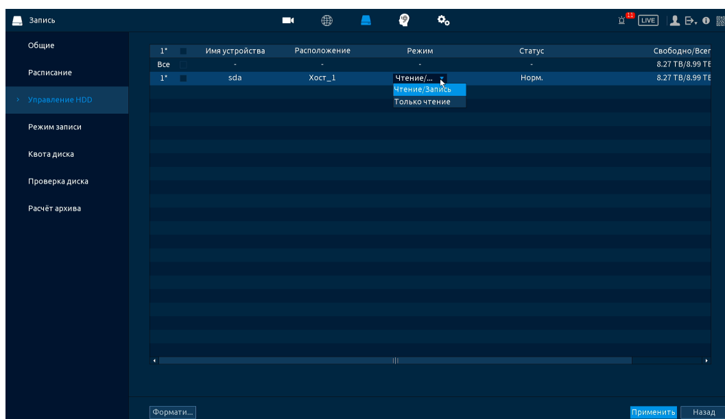
Рисунок 13.15 – Интерфейс настройки
