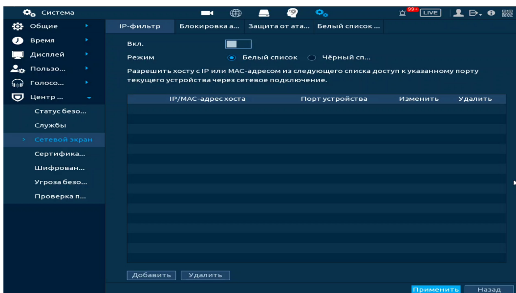
Рисунок 17.42 – Сетевой экран
