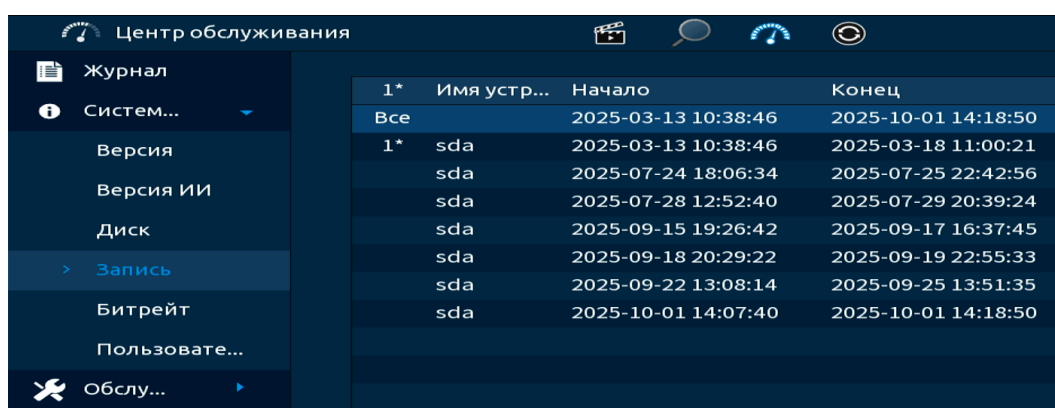
Рисунок 18.5 – Интерфейс просмотра
