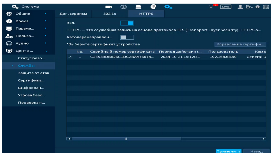
Рисунок 17.39 – HTTPS
