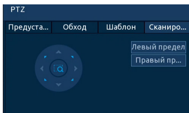
Рисунок 9.11 – Интерфейс «Сканирование»
