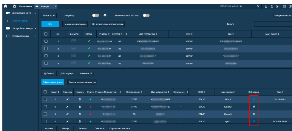
Рисунок 21.4 – Список камер
