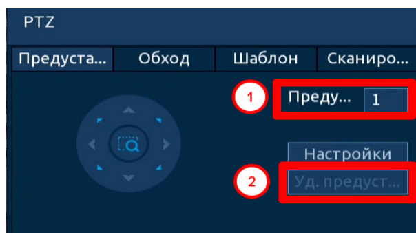
Рисунок 9.7 – PTZ предустановка
