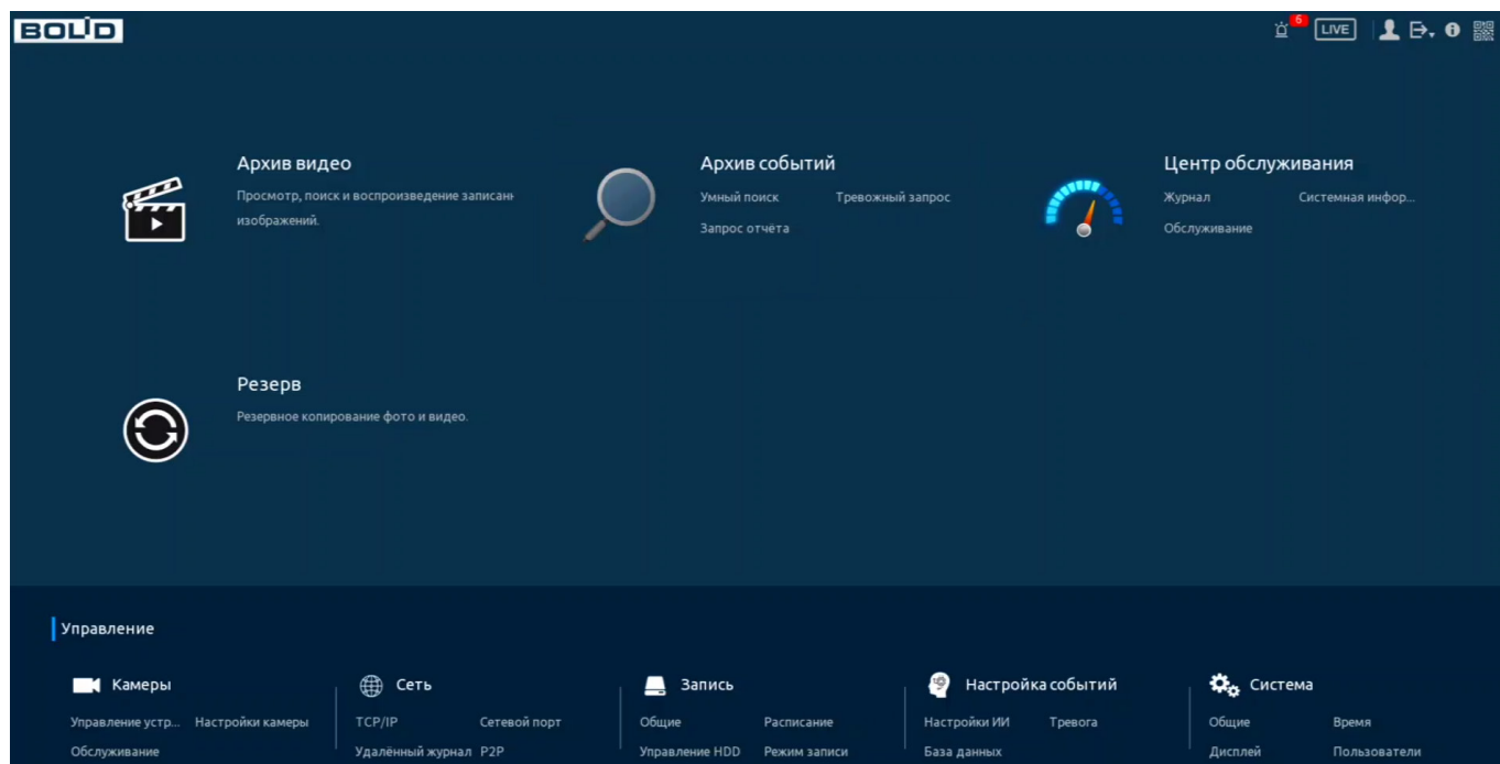
Рисунок 10.1 – Главное меню
