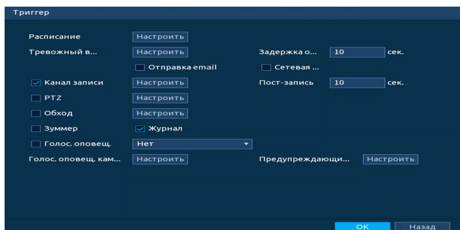
Рисунок 14.64 – Настройка параметров
