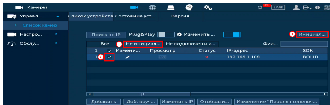
Рисунок 11.11 – Инициализация устройства
