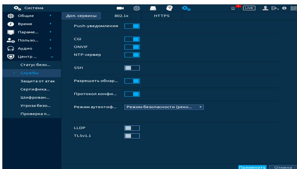
Рисунок 17.36 – Системное обслуживание
