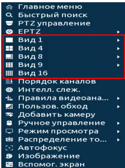
Рисунок 8.1 – Контекстное меню
