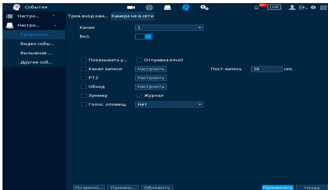
Рисунок 14.5 – Интерфейс настройки
