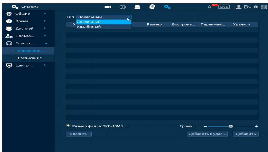
Рисунок 17.29 – Управление файлами
