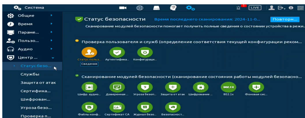
Рисунок 17.35 – Статус безопасности
