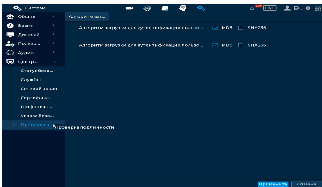
Рисунок 17.58 – Безопасная аутентификация
