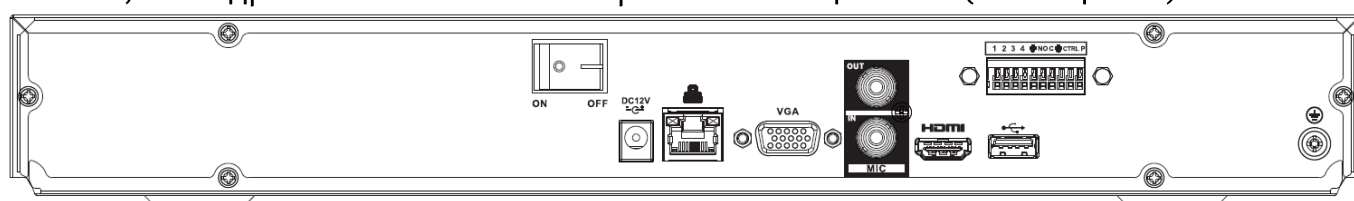
Рисунок 1.7 – Внешний вид задней панели корпуса
