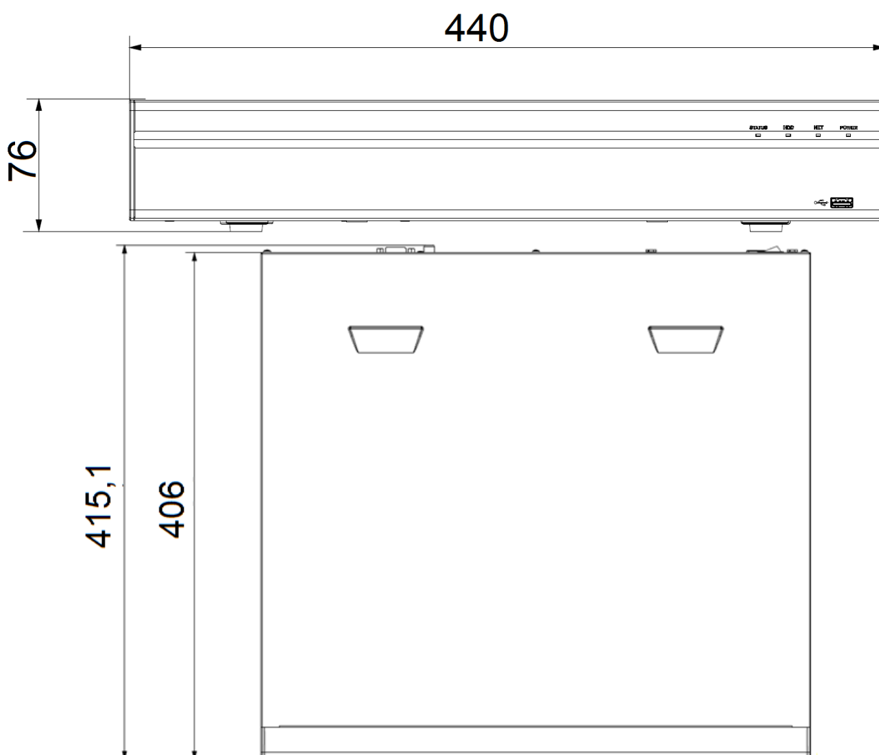
Рисунок 4.1 – Габаритные размеры видеорегистратора
