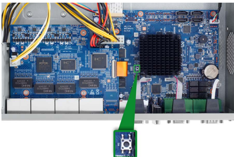
Рисунок 26.8 – Пример расположения кнопки сброса
