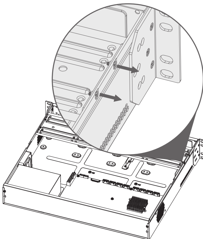
Рисунок 4.4 – Установка жёсткого диска
