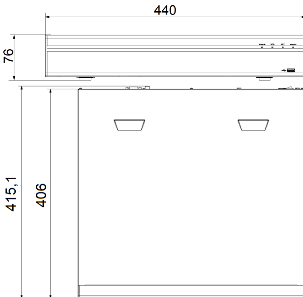
Рисунок 4.1 – Габаритные размеры видеорегистратора
