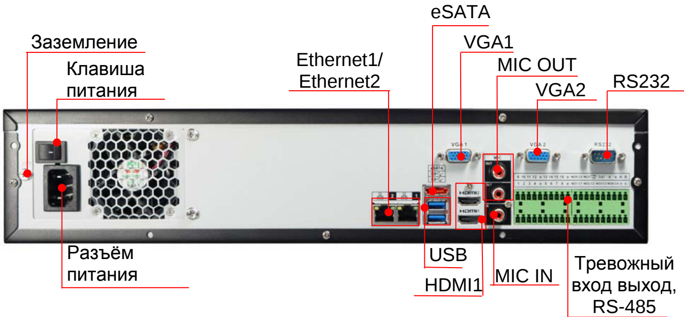
Рисунок 3.2 – Внешний вид задней панели корпуса
