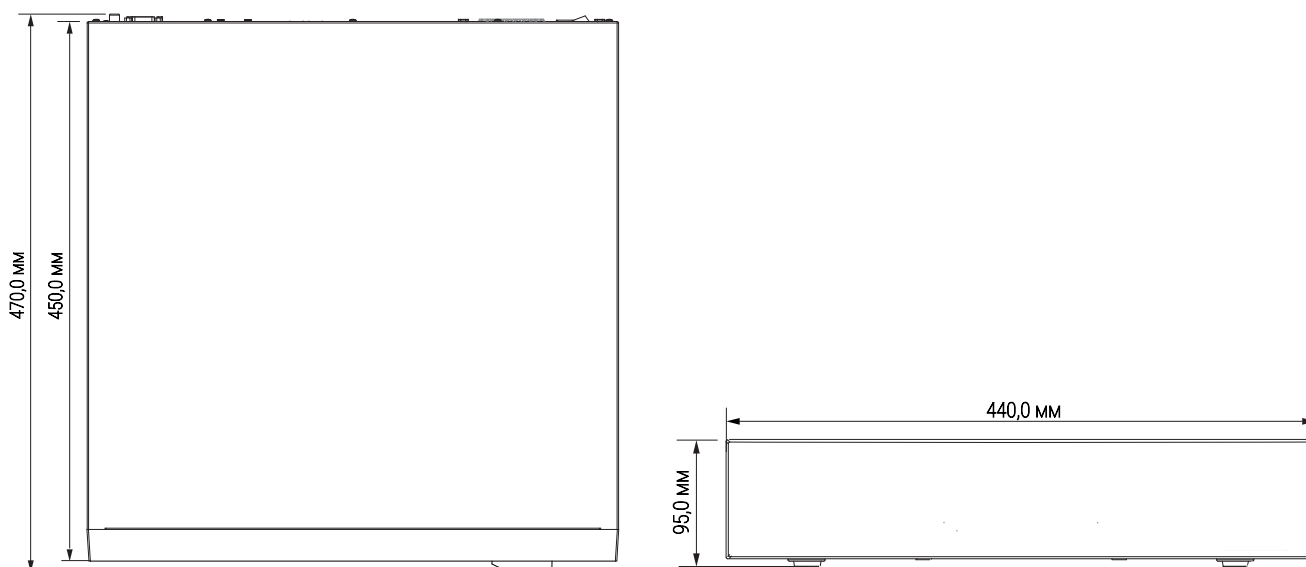
Рисунок 4.1 – Габаритные размеры видеорегистратора
