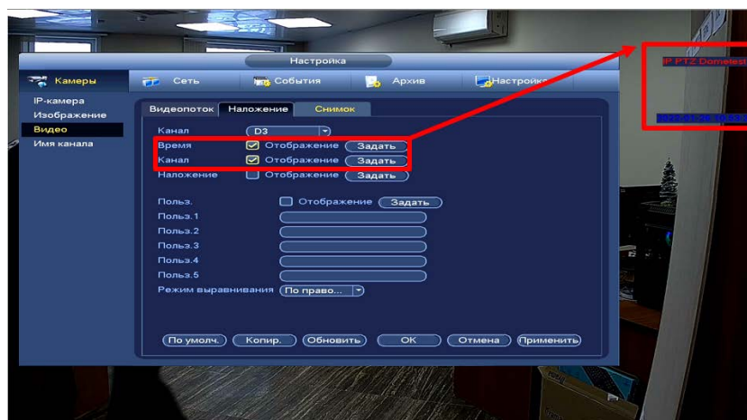
Рисунок 15.6 – Наложенные параметры
