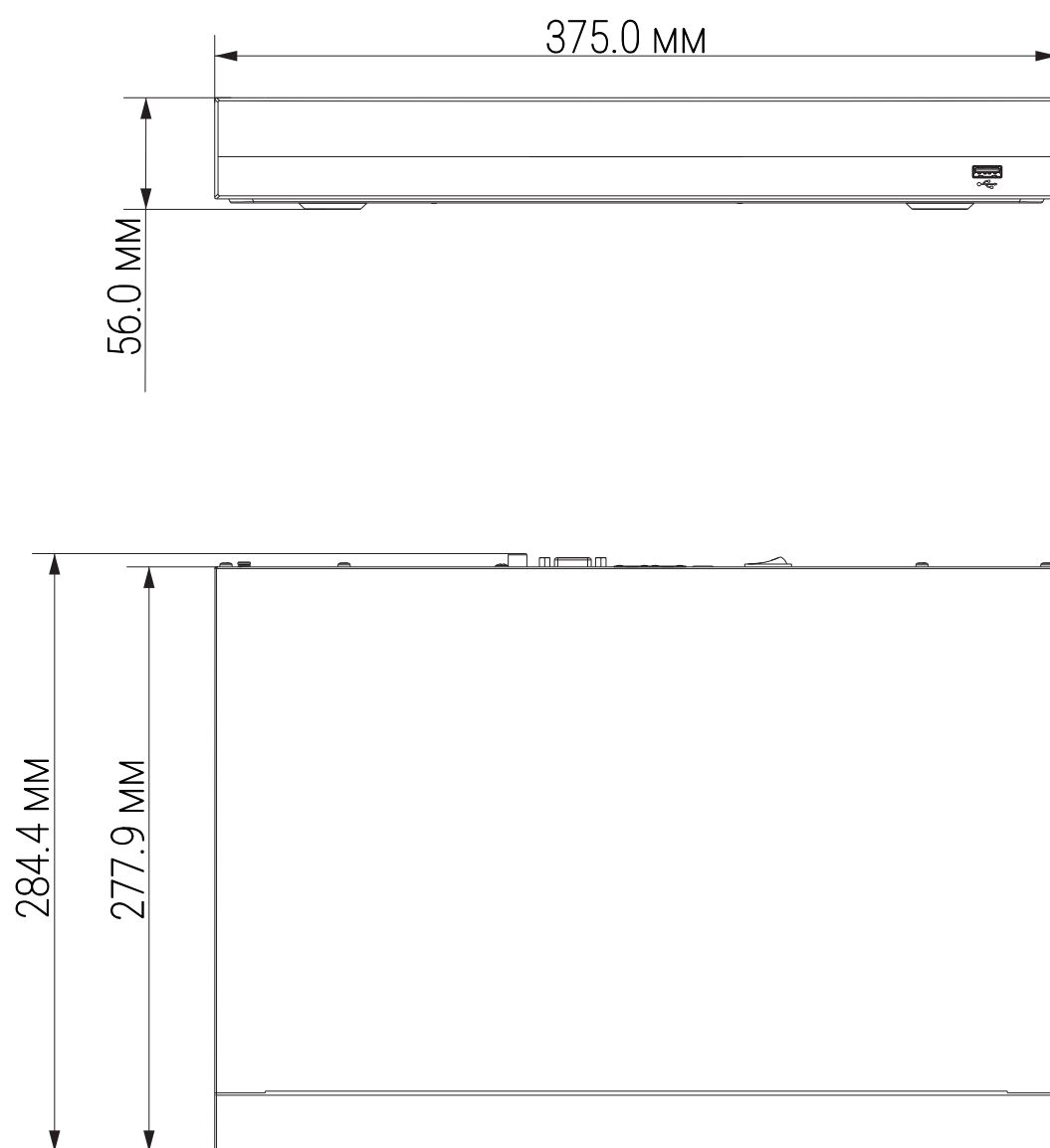
Рисунок 4.1 – Габаритные размеры видеорегистратора
