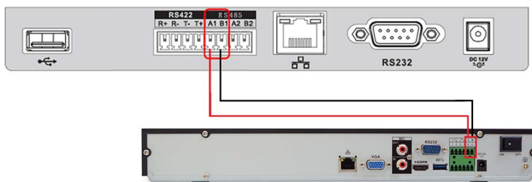
Рисунок 15.4 – Схема RS-485
