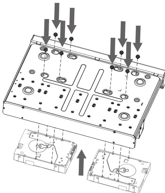
Рисунок 4.4 – Установка жёсткого диска
