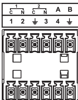
Рисунок 3.3 – Тревожный вход/выход, RS-485
