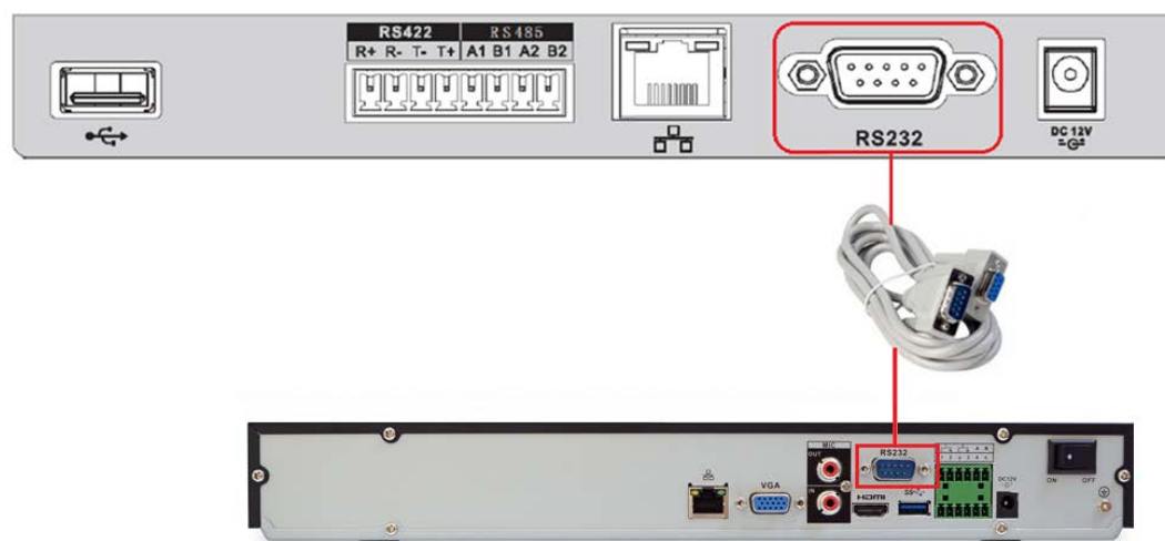
Рисунок 15.5 – Схема RS-232
