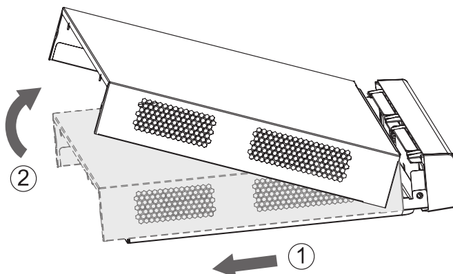
Рисунок 4.3 – Установка жёсткого диска
