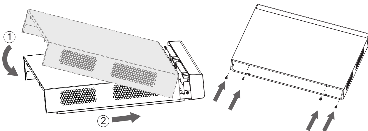
Рисунок 4.6 – Установка жёсткого диска
