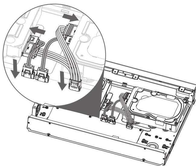
Рисунок 4.5 – Установка жёсткого диска
