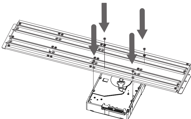
Рисунок 4.5 – Установка жёсткого диска
