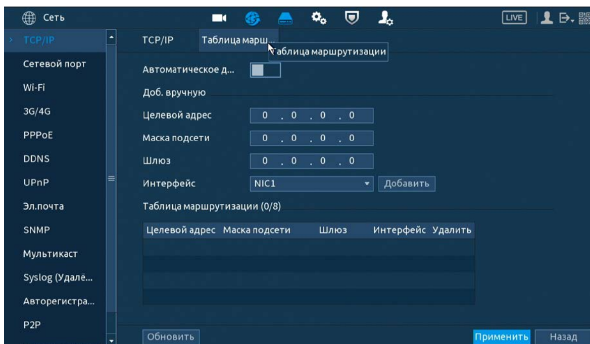
Рисунок 13.3 – Интерфейс настройки «Таблица маршрутизации»
