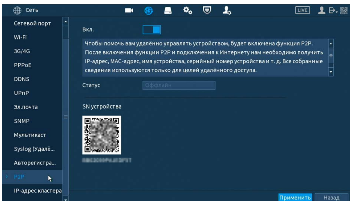
Рисунок 13.17 – Интерфейс включения «P2P»
