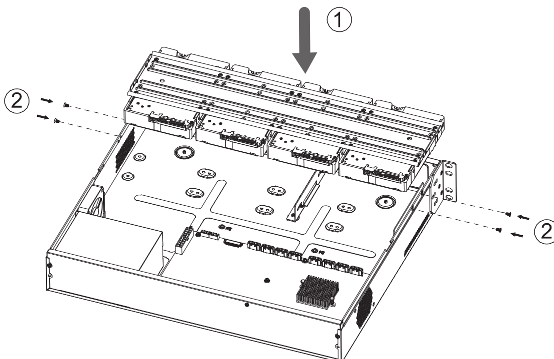
Рисунок 4.6 – Установка жёсткого диска
