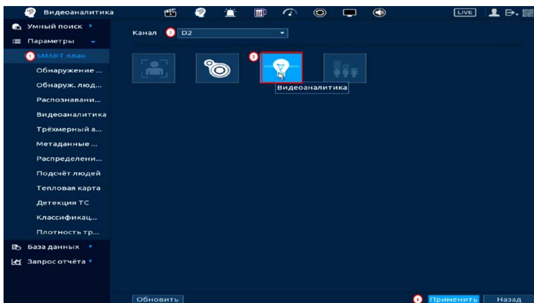
Рисунок 20.69 – Настройка
