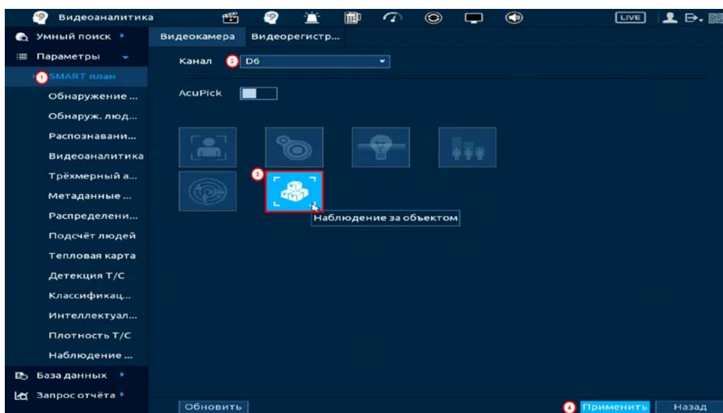
Рисунок 20.139 – Настройка
