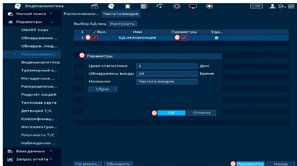
Рисунок 20.33 – Настройка
