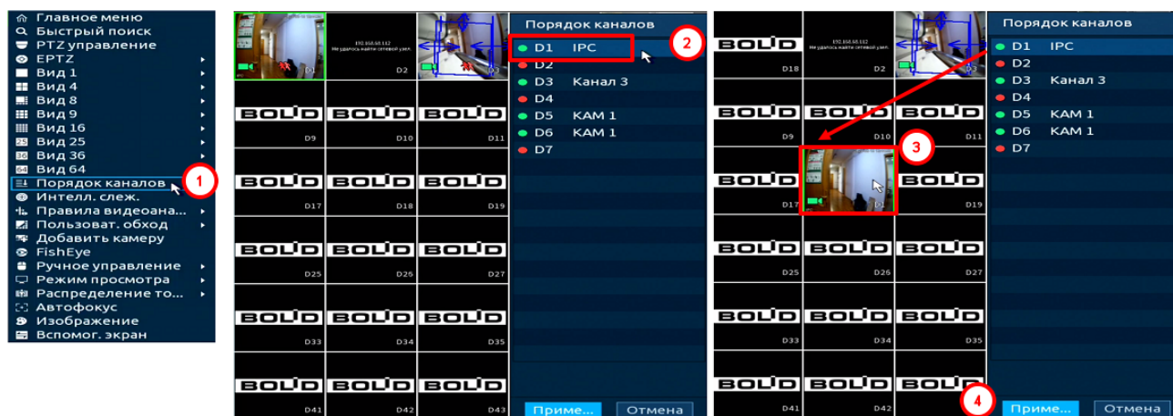
Рисунок 8.6 – Изменение раскладки
