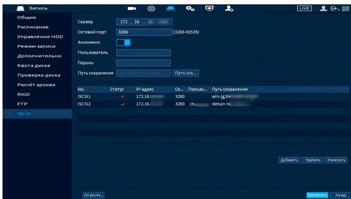
Рисунок 14.33 – Настройка iSCSI
