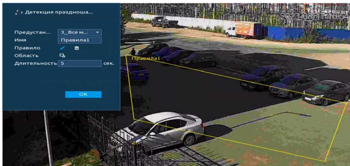
Рисунок 20.83 – Настройка правила
