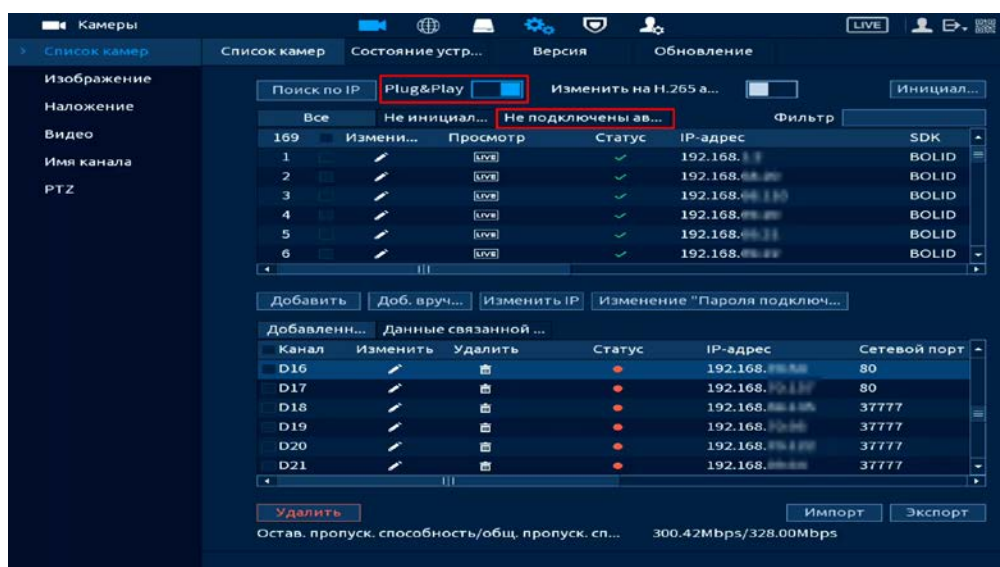
Рисунок 12.6 – Plug&Play
