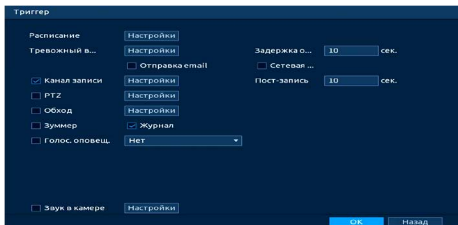
Рисунок 20.54 – Настройка
