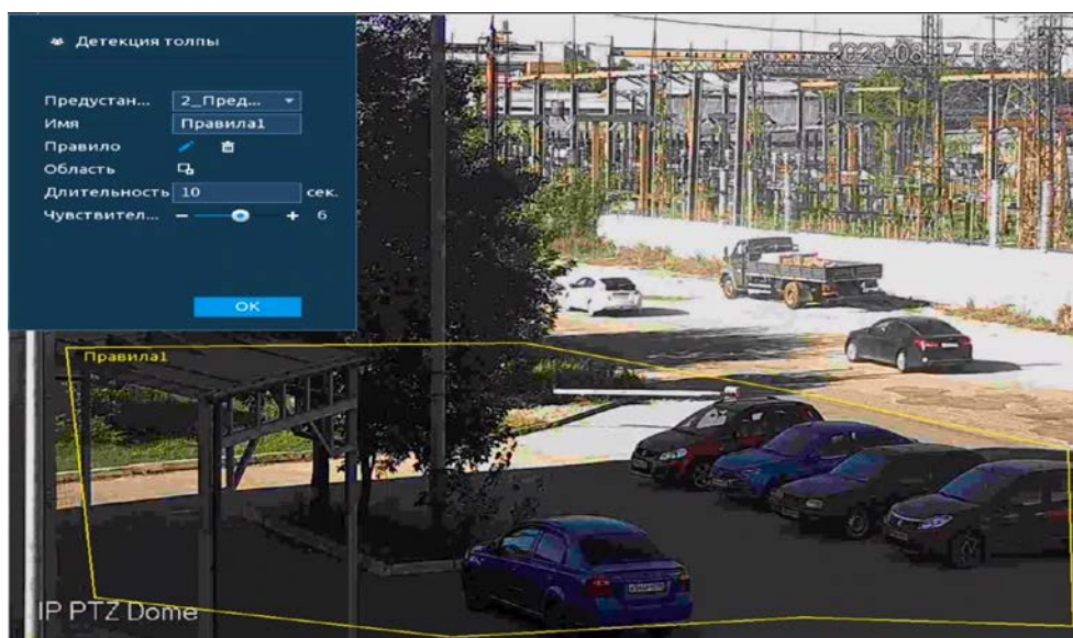
Рисунок 20.77 – Настройка правила
