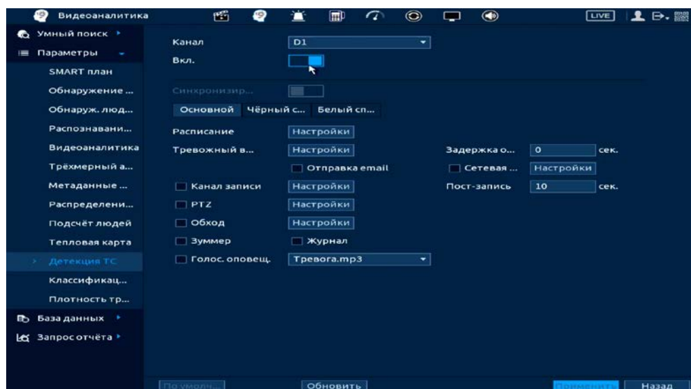
Рисунок 20.123 – Настройка детекции
