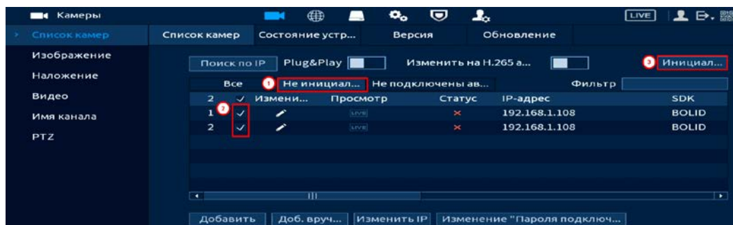
Рисунок 12.10 – Инициализация устройства
