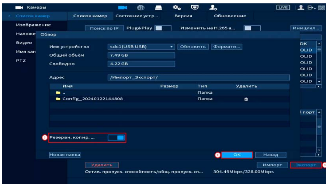
Рисунок 12.22 – Экспорт
