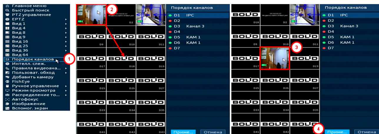
Рисунок 8.7 – Изменение раскладки
