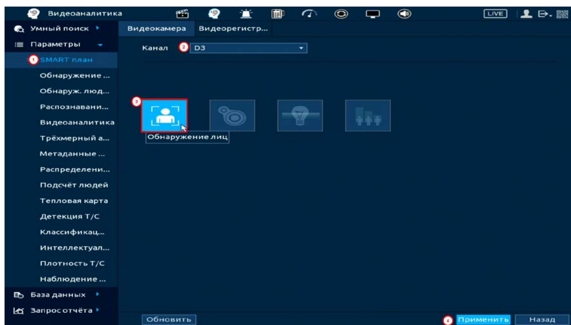
Рисунок 20.14 – Настройка
