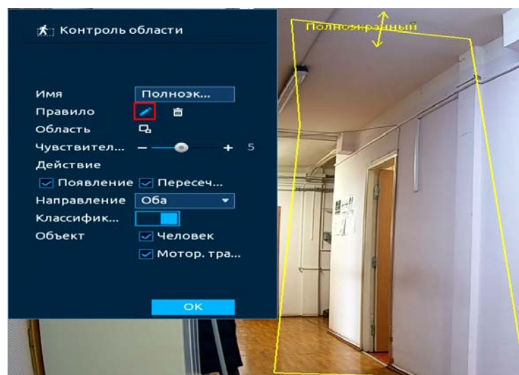
Рисунок 20.45 – Настройка
