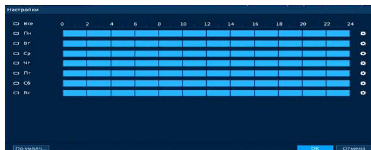
Рисунок 20.61 – Расписание
