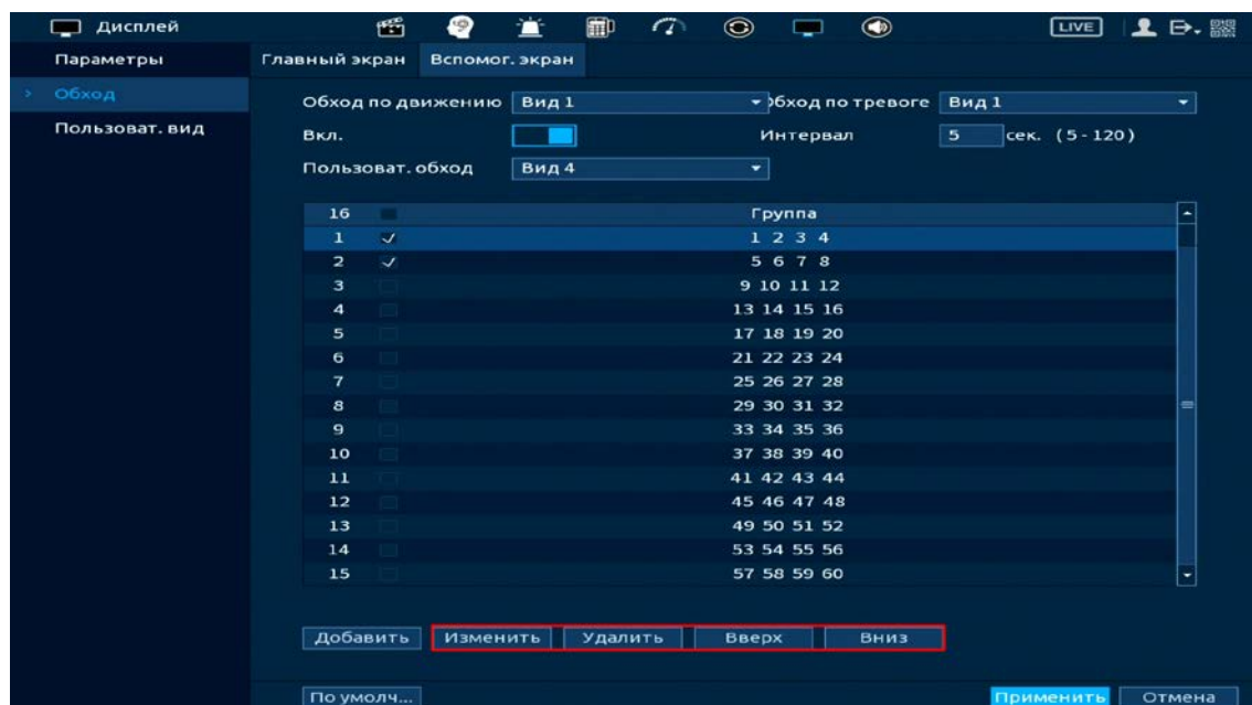
Рисунок 10.12 – Расположение групп
