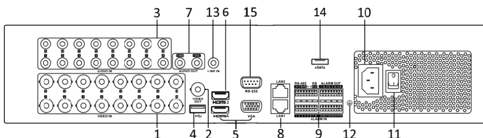
Рисунок 1-9 Задняя панель DS-8100HUNI-F8/N
