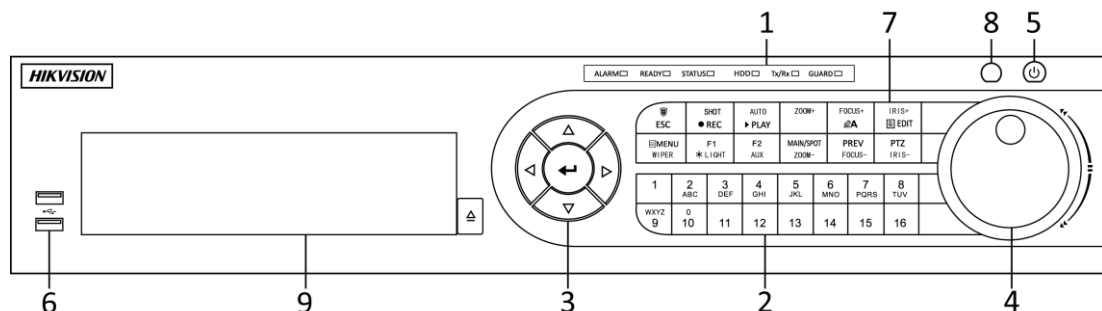
Рисунок 1-4 Передняя панель DS-8100HQHI-F/N и DS-8100HUNI-F/N
