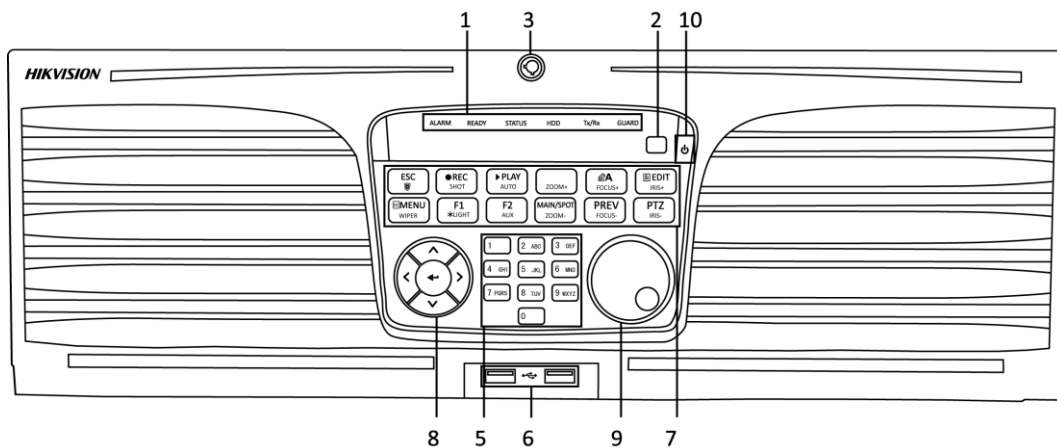
Рисунок 1-6 Передняя панель DS-9000HUNI-F16/N
