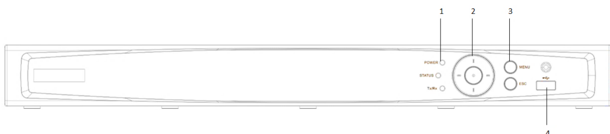
Рисунок 1-2 Панель DS-7200HGHI/ DS-7200HQHI-F/N/ DS-7200HUI-F/N и DS-7600HUI-F/N
