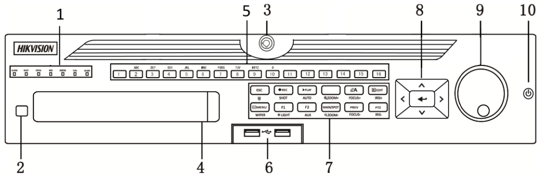
Рисунок 1-5 Передняя панель DS-9000HUNI-F8/N
