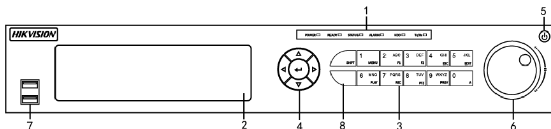
Рисунок 1-3 Передняя панель DS-7300HQHI-F/N и DS-7300HUNI-F/N
