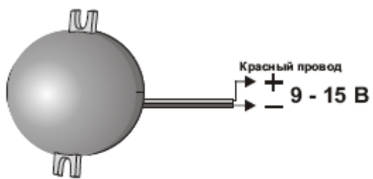
Рис.2 Схема подключения ПКИ - СО1(И).
