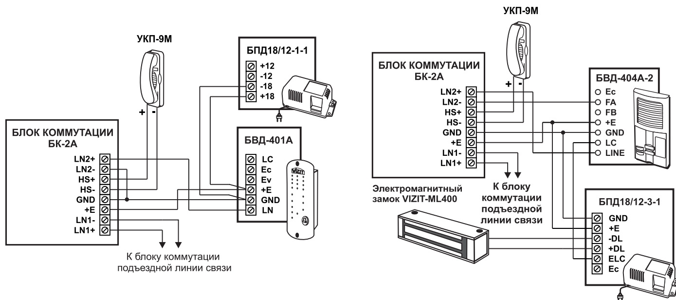
Рисунок 1. Схемы соединений УКП с подъездным и этажным блоками вызова с использованием блока коммутации БК-2А.
