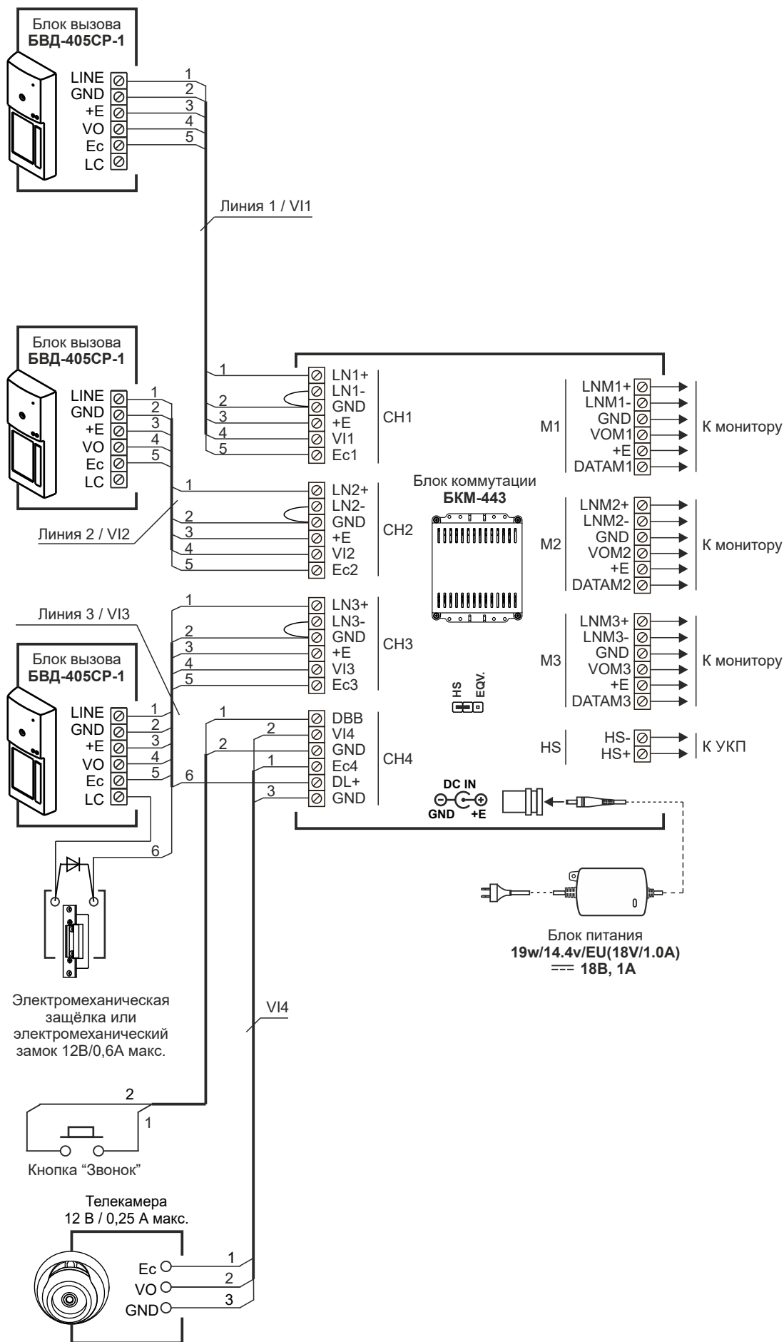
Схема соединений блока коммутации БКМ-443(С) с тремя блоками вызова БВД-405СР-1 и блоком БВД-403СРО (телекамера + кнопка “Звонок”)
