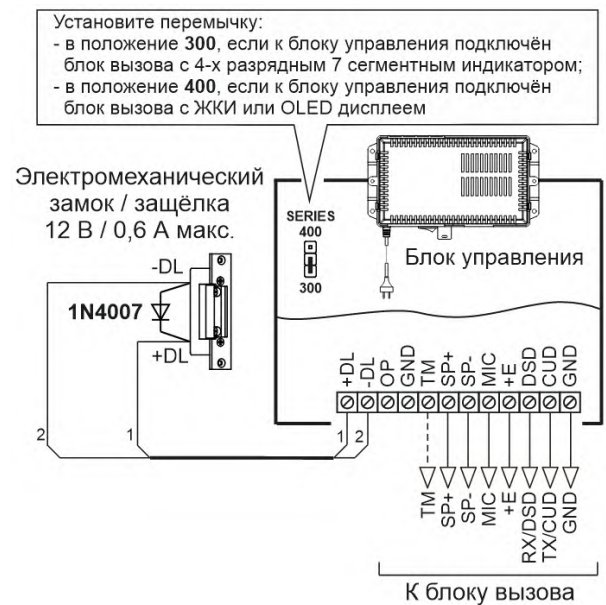
Рисунок 11.4 – Схема соединений блока управления, блока вызова и электромеханического замка / защёлки
