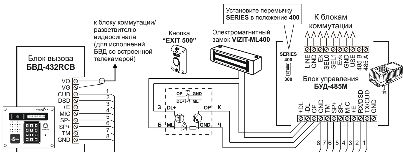
Рисунок 9 - Схема соединений блока вызова БВД-432RCB с блоком управления БУД-485М , электромагнитным замком VIZIT-ML400 и кнопкой “EXIT 500”
