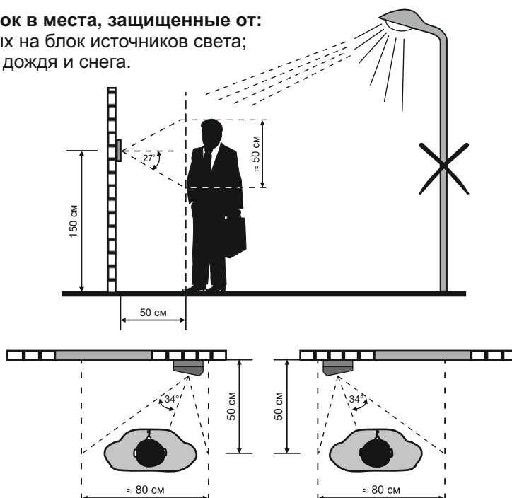
Рисунок 5 - Рекомендуемая высота установки блока и область обзора тепекамеры
