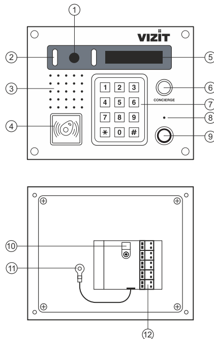
Рисунок 1 - Внешний вид блока
