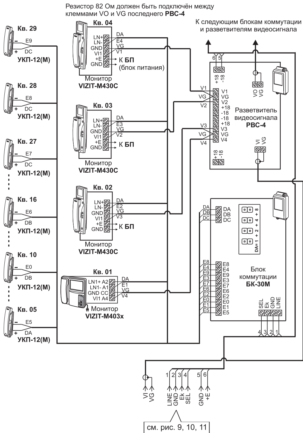
Рисунок 20 - Схема соединений блока вызова БВД-SM101RCPL(TCPL) с блоками коммутации БК-30М , разветвителями видеосигнала РВС-4 , мониторами и УКП в составе видеодомофона
