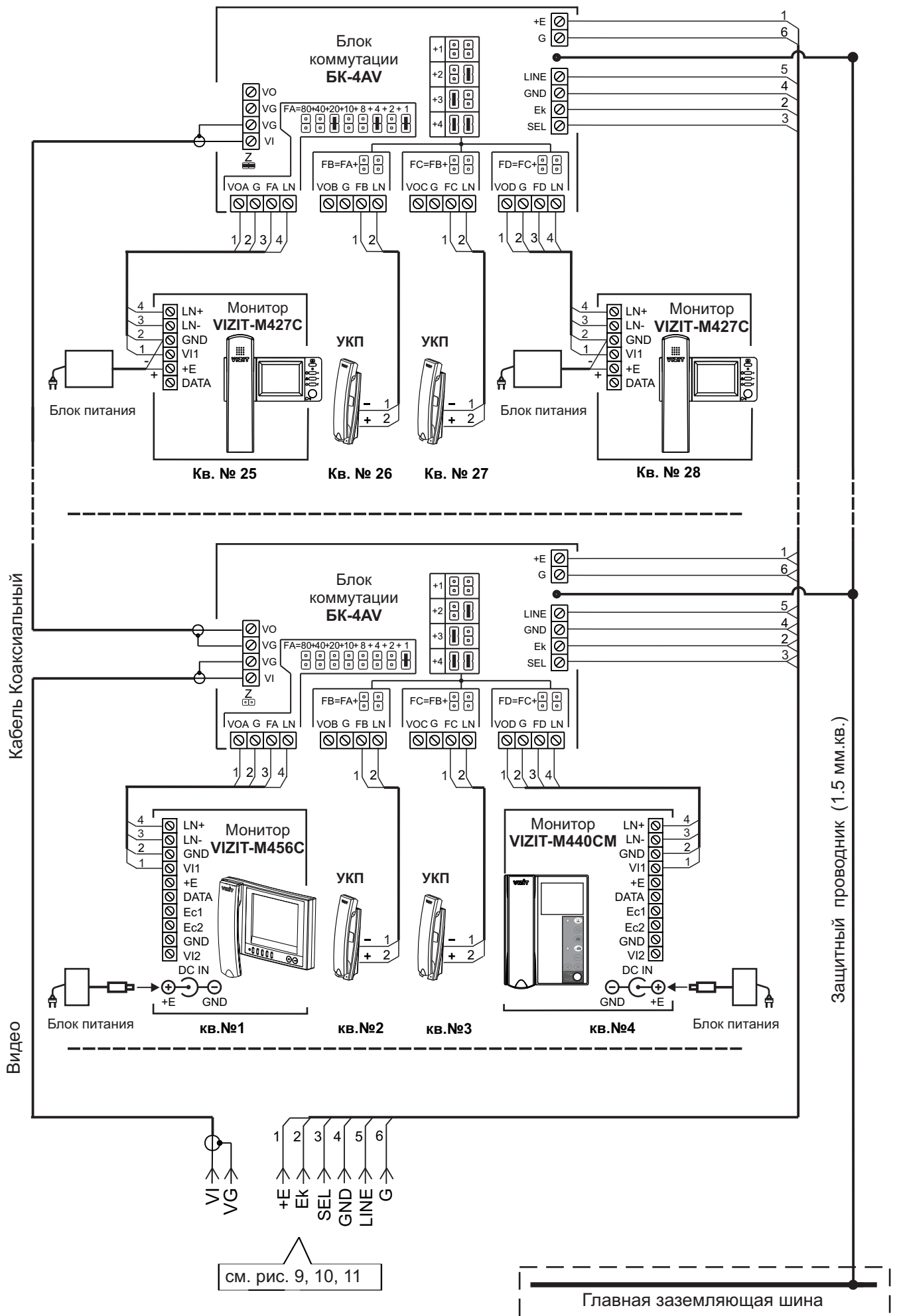
Рисунок 17 - Схема соединений блока вызова БВД-SM110FCP с блоками коммутации БК-4АВ и мониторами VIZIT в составе многоабонентского видеодомофона до 100 абонентов
