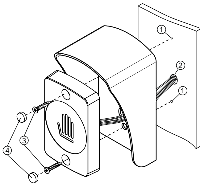
Крепление кнопки на неподвижную часть металлической двери с использованием монтажного комплекта MK-RD
