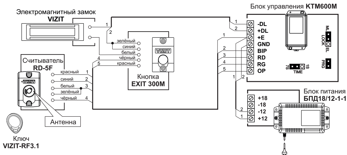
Контроллер с электромагнитным замком и кнопкой EXIT 300M
