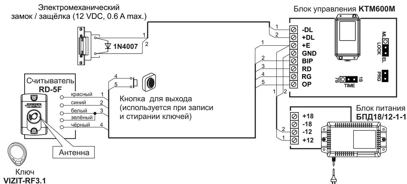
Контроллер с электромеханическим замком
