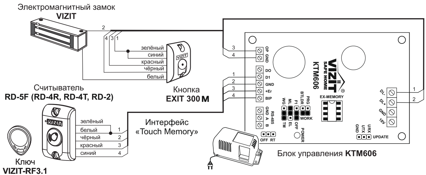
Контроллер с электромагнитным замком и кнопкой EXIT 300M
