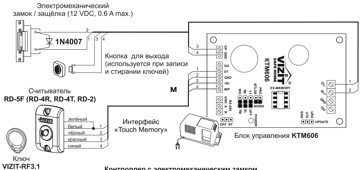
Контроллер с электрохимическим замком
