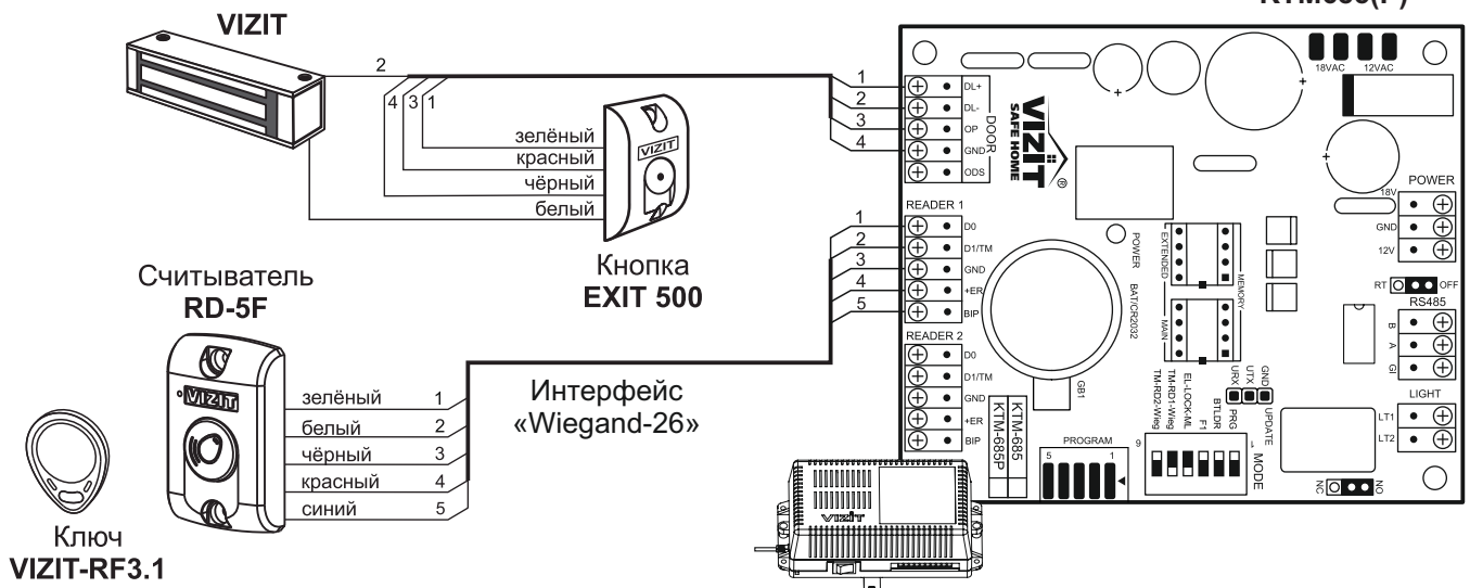
Контроллер с электромагнитным замком и кнопкой EXIT 500
