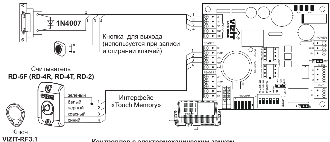
Контроллер с электромеханическим замком
