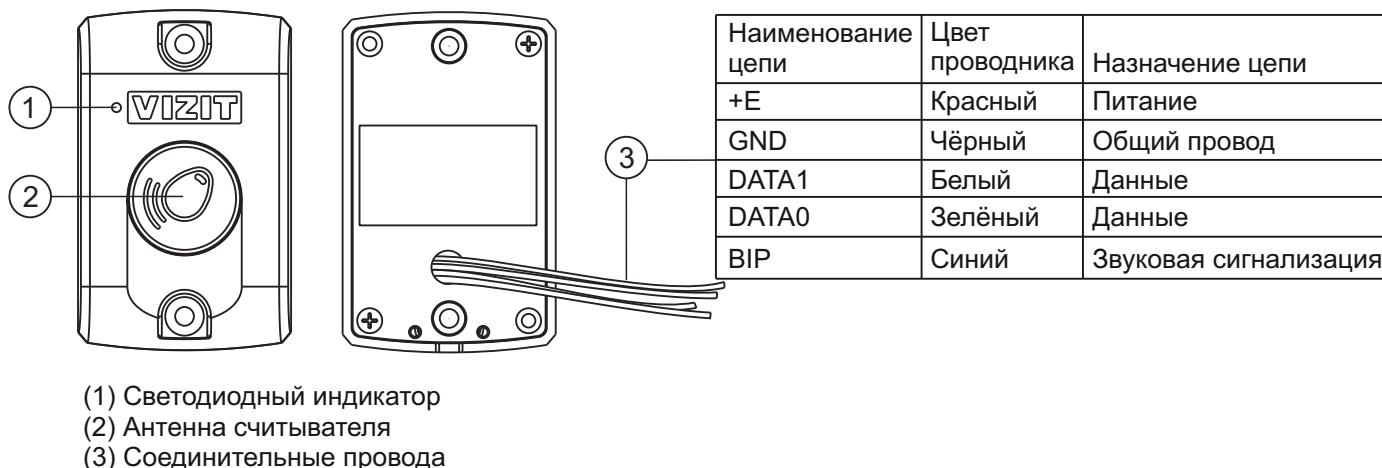
Внешний вид считывателя RD-5F, наименование цепей и их назначение
