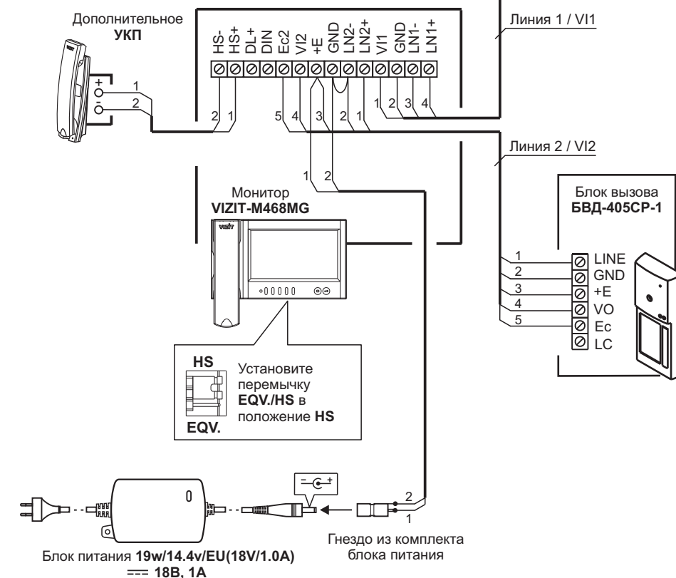
Схема соединений монитора с блоком коммутации подъездного / многоабонентского видеодомофона, блоком вызова на 1 абонента и дополнительным УКП
