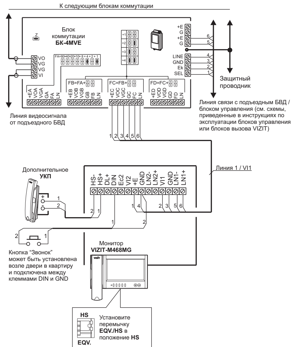
Схема соединений монитора с блоком коммутации подъездного / многоабонентского видеодомофона, дополнительным УКП и кнопкой "Звонок". Питание монитора обеспечивается от группового блока питания.
