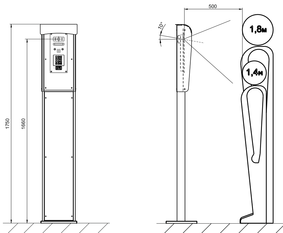
Рис.9 Установлен БВД-440FCBE/740FCBE (диагональ объектива телекамеры - 92°)
