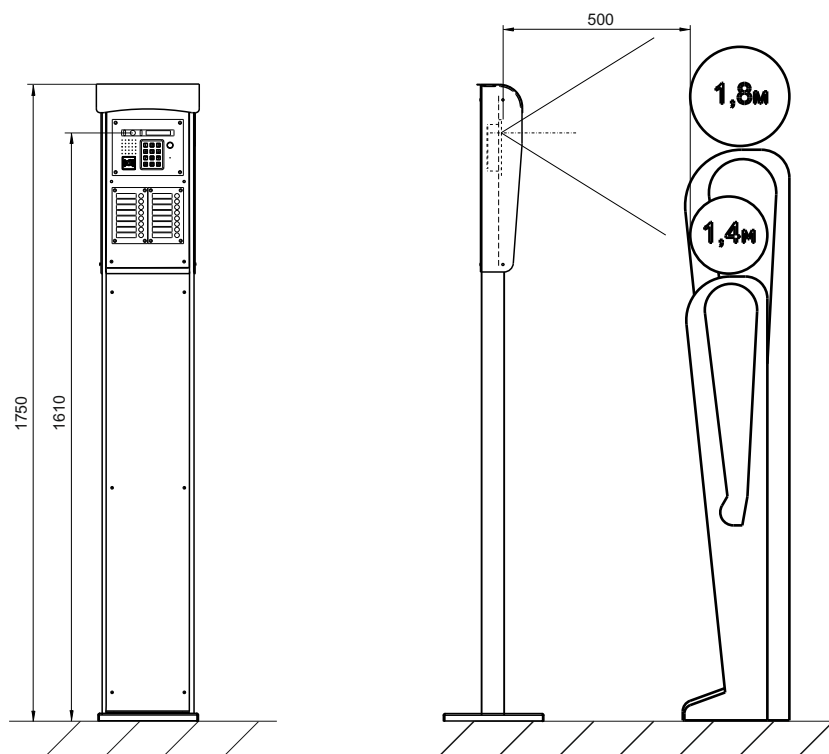
Рис.7 Установлен БВД-533FCBE/733FCBE (диагональ объектива телекамеры - 92°)
