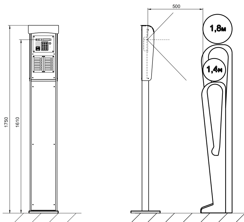
Рис.6 Установлен БВД-432FCB/532FCB (диагональ объектива телекамеры - 120°)
