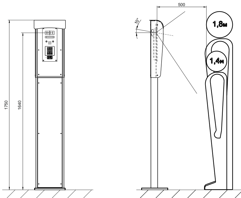
Рис.8 Установлен БВД-440FCВ (диагональ объектива телекамеры - 120°)
