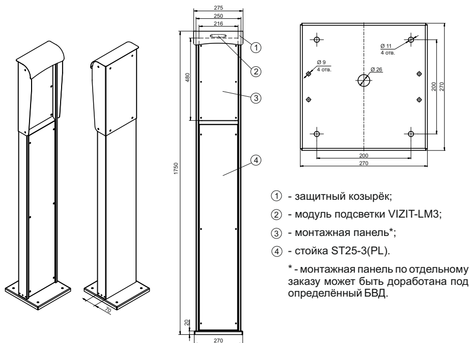
Рис.2 Внешний вид, габаритные и установочные размеры стойки ST25-3(PL)
