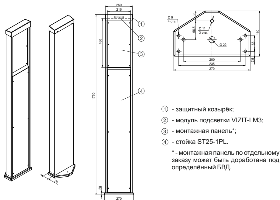
Рис.1 Внешний вид, габаритные и установочные размеры стойки ST25-1PL
